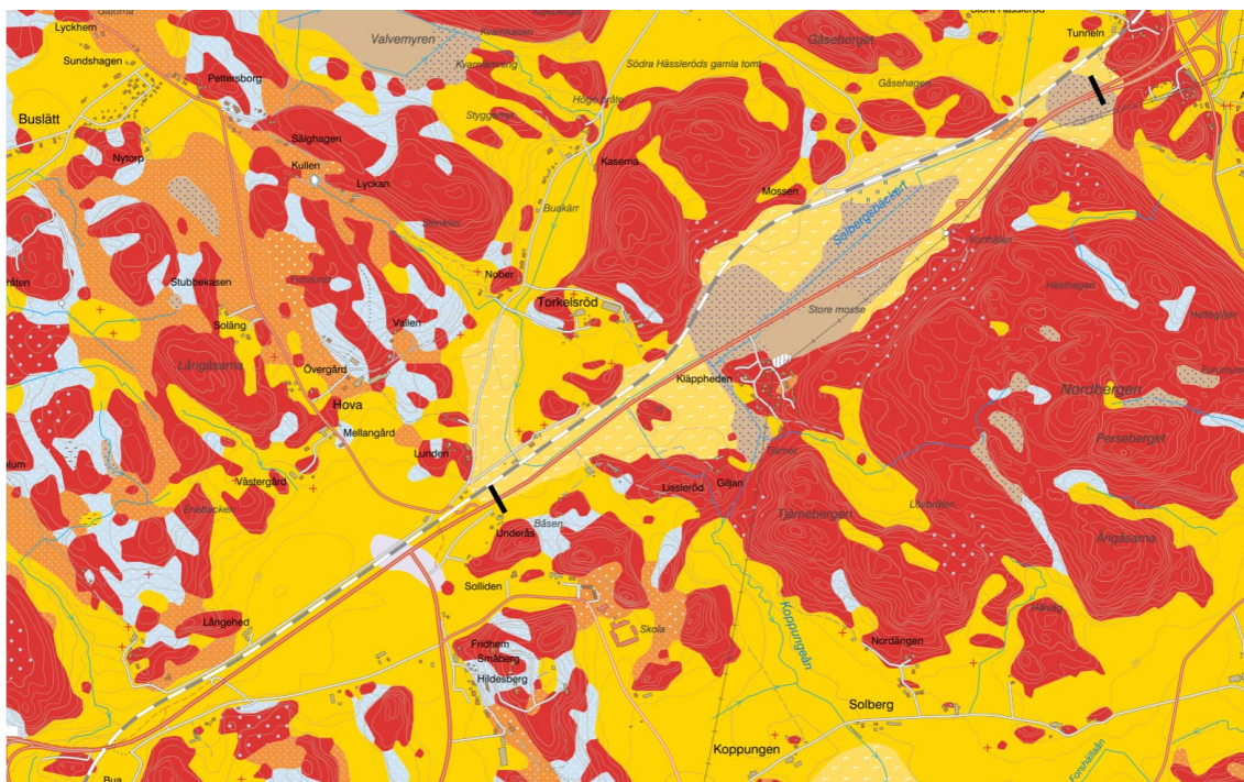
Figur 26. Jordartskarta från SGU med jordarter i närheten av markytan. Ungefärlig aktuell sträcka mellan de svarta markeringarna.
