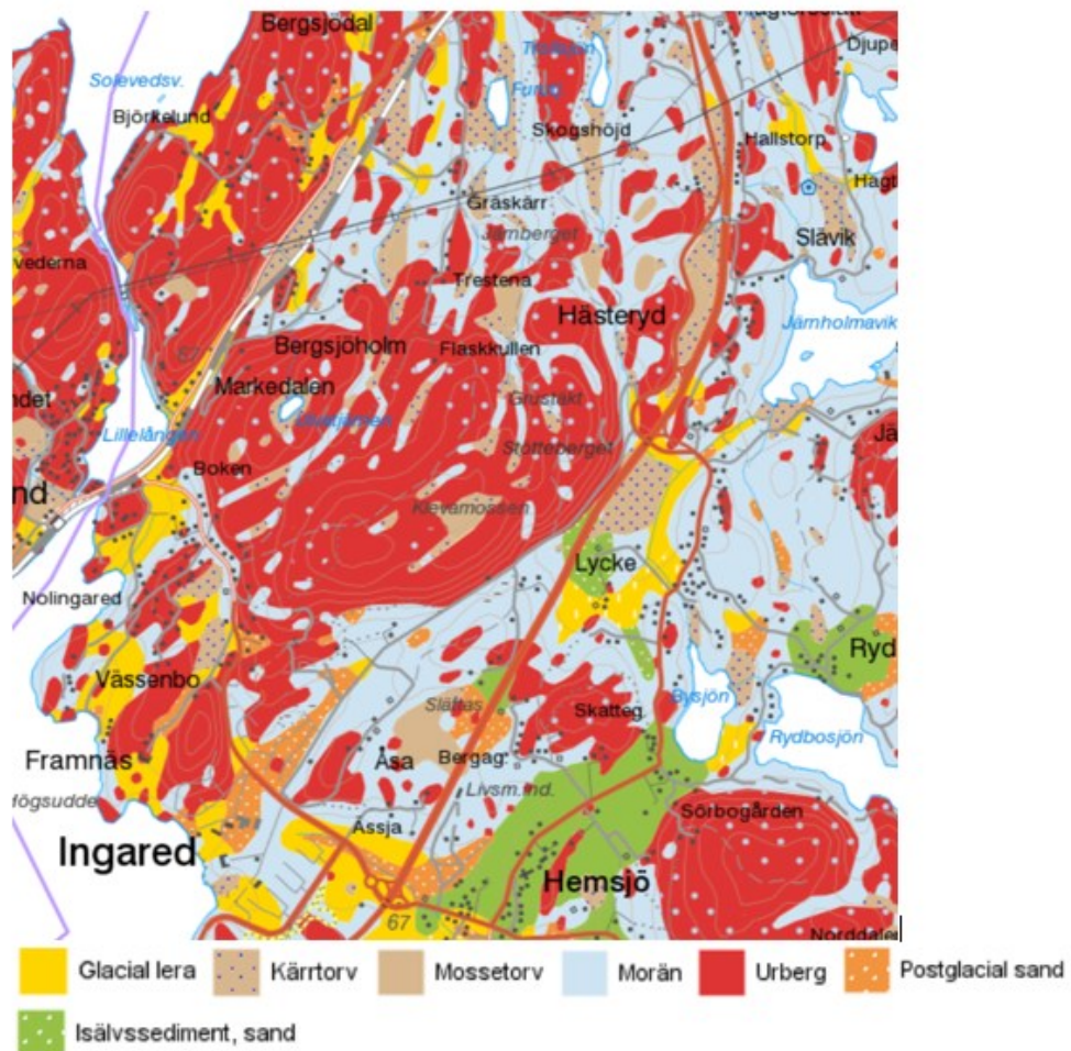
Figur 20. Utsnitt ur SGU:s jordartskarta över yttliga jordarter.
