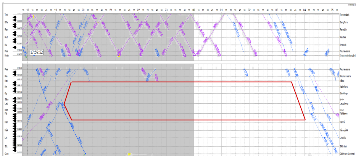
Figur 11: Spårbytets arbetsperiod i den grafiska tidtabellen
