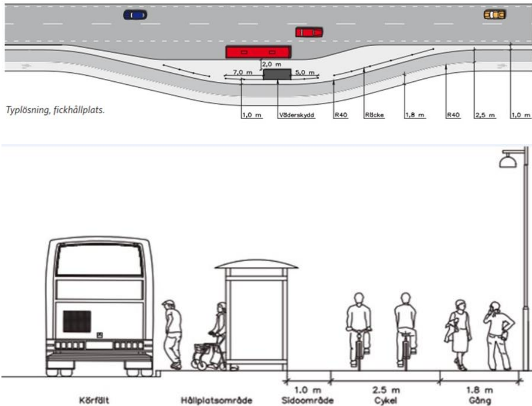
Bild 30. Princip för utformning vid busshållplatser (Källa: regional cykelplan för Stockholms län).
