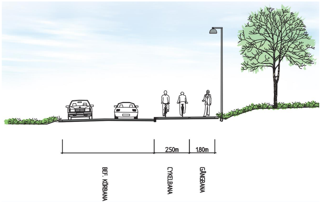
Bild 25. Kantstensförlagd GC-väg utan skiljeremsa.
