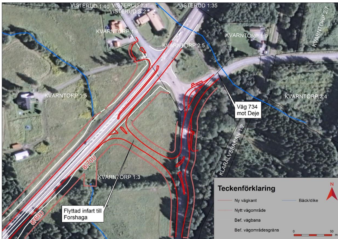
Figur 22. Norra infarten till Forshaga flyttas knappt 100 meter söderut för att skapa en trafiksäker lösning.
