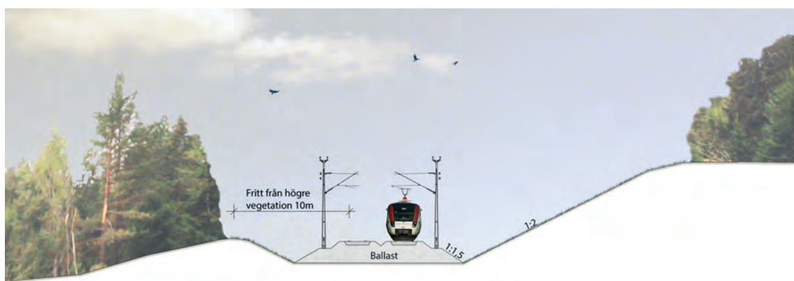
Figur 6.2-4. Illustration av järnväg i jordskärning i skogslandskap.
