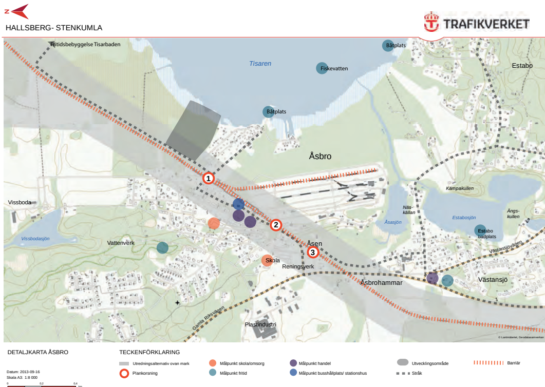
Figur 3.5-3 Befintliga plankorsningar och målpunkter i Åsbro
