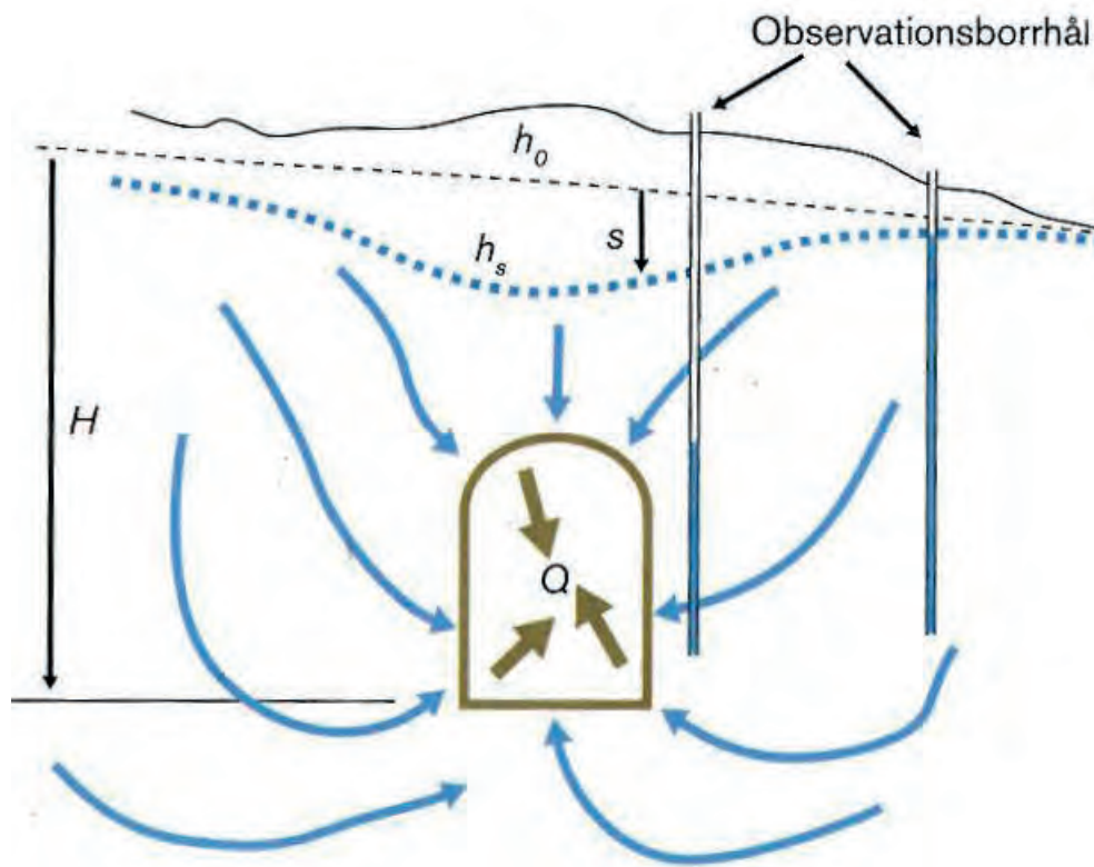
Figur 7.3-8 Grundvattenströmning intill en tunnel. Bilden representerar en otätad tunnel och hur grundvattensänkning ovan tunneln kan se ut. Även med tätningsåtgärder brukar tunnlar dock aldrig bli helt täta. Dessutom har jordarternas genomsläpplighet och spricksystemens utbredning och storlek betydelse för hur stor sänktratten blir ovanför tunneln och hur grundvattensänkning utbreder sig.
