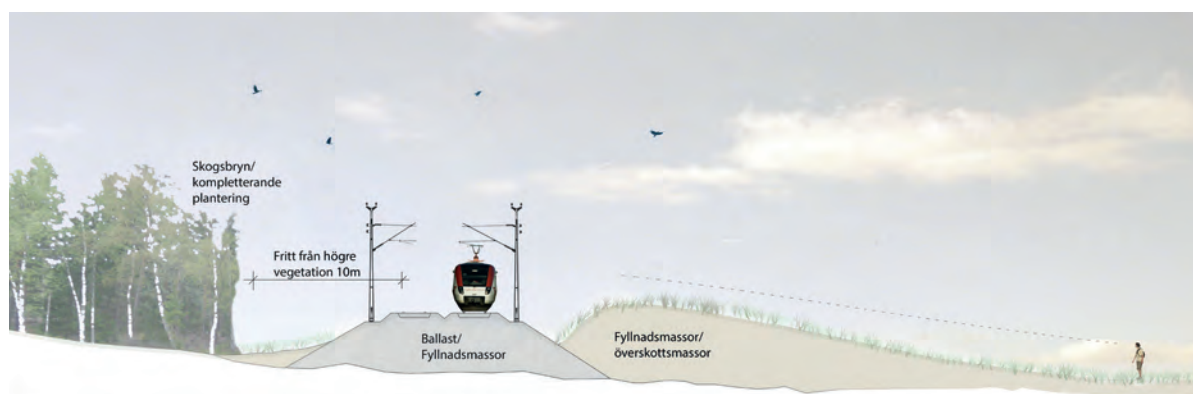
Figur 6.2-2. Vid områden där järnvägen upplevs som en stor störning kan dess påverkan minskas med hjälp av terrängmodellering och/eller kompletterande plantering. Järnväg bör om möjligt förläggas vid skogsbryn för att minimera fragmentering av öppna landskap.
