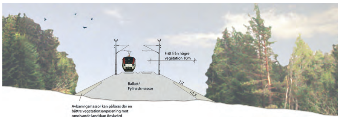
Figur 6.2-3. Illustration av järnväg på hög bank med brantare släntlutning i skogsmark.
