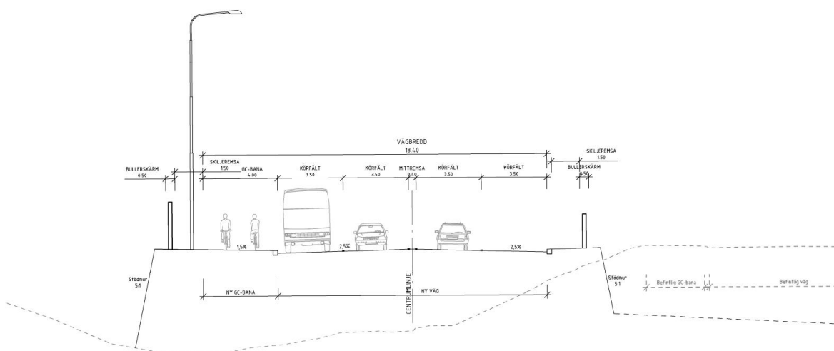
Figur 3.4 Vägsektion sträckan Tappsström till Färentunavägen, vy sedd från Ekerö
