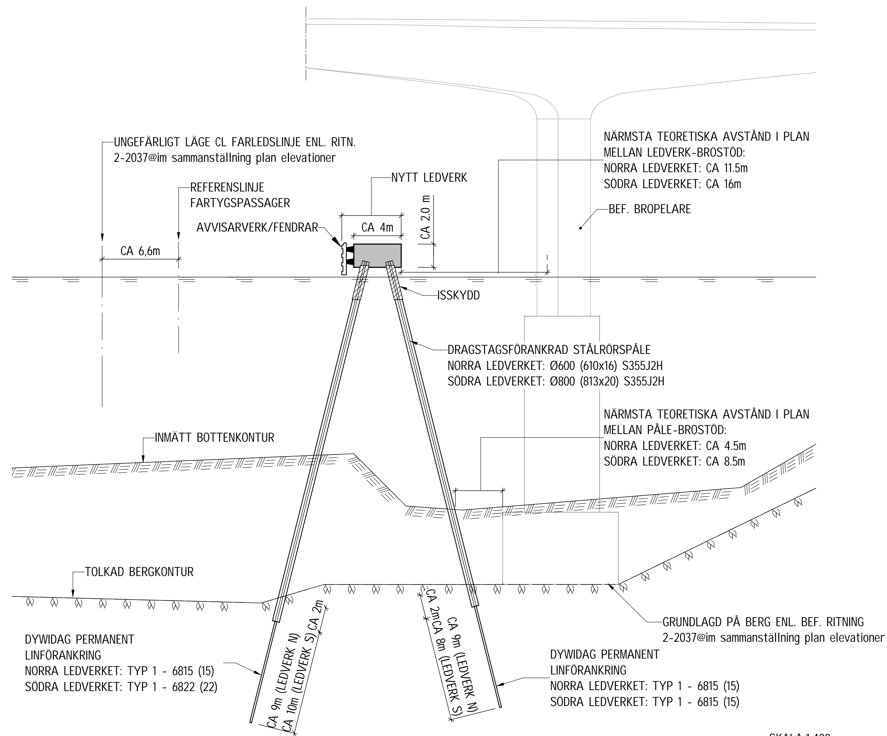
SEKTION B-B 1 : 200
