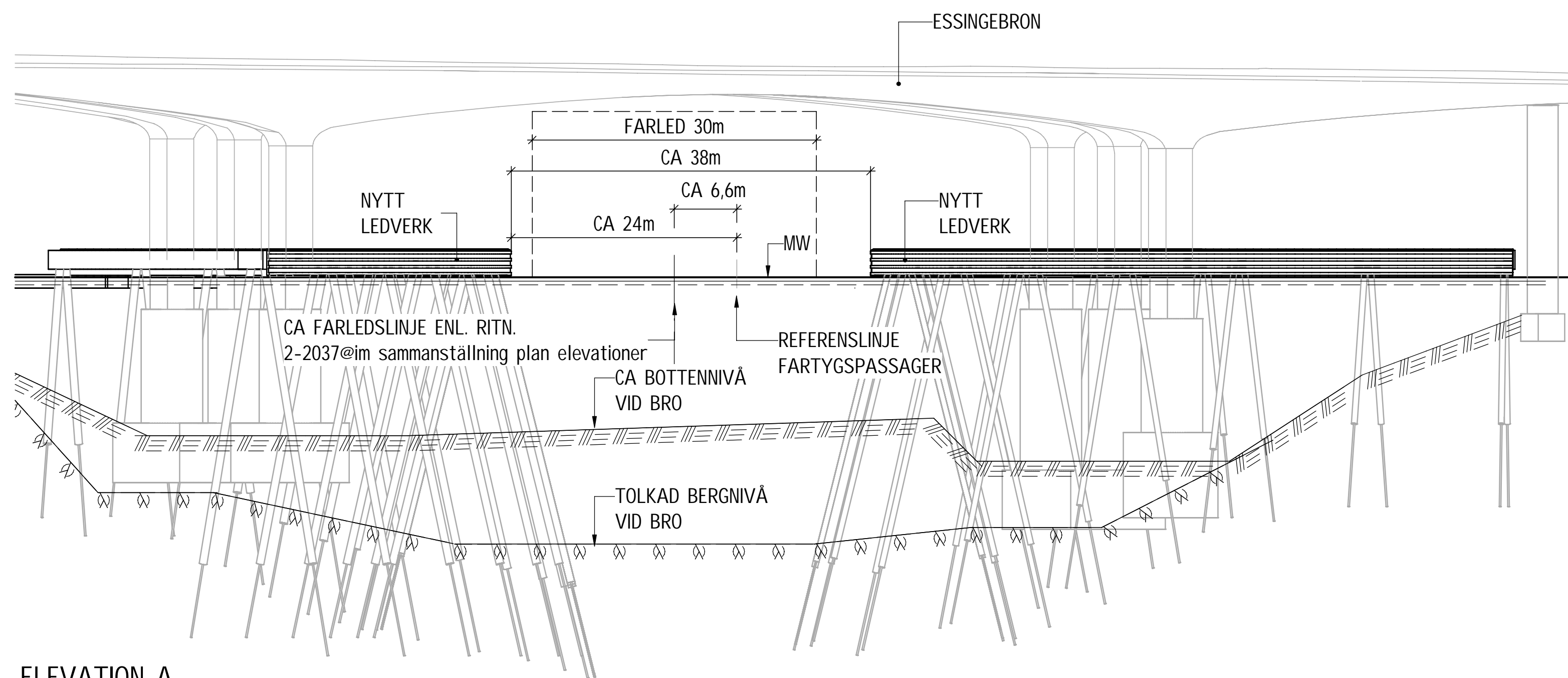
ELEVATION A 1 : 400
