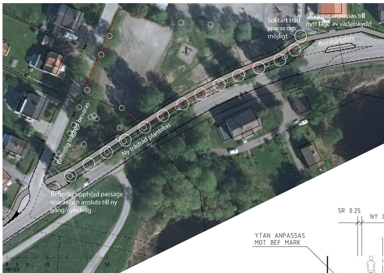
Figur 8. Plan över gång- och cykelväg förbi skolan med ny trädrad i skiljeremsa.
