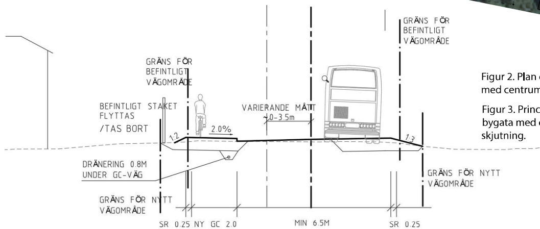
Bild 7. Läge där centrumlinje förskjuts och vägbana breddas till vänster i bild.
