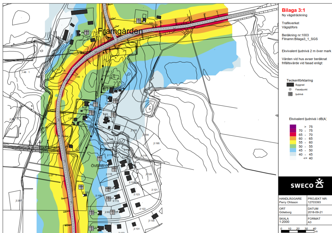
Figur 17. Bullerberäkning av ekvivalent ljudnivå i alternativ N.
