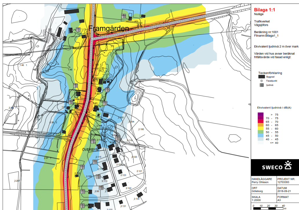
Figur 11. Bullerberäkning av ekvivalent ljudnivå i nuläget.
