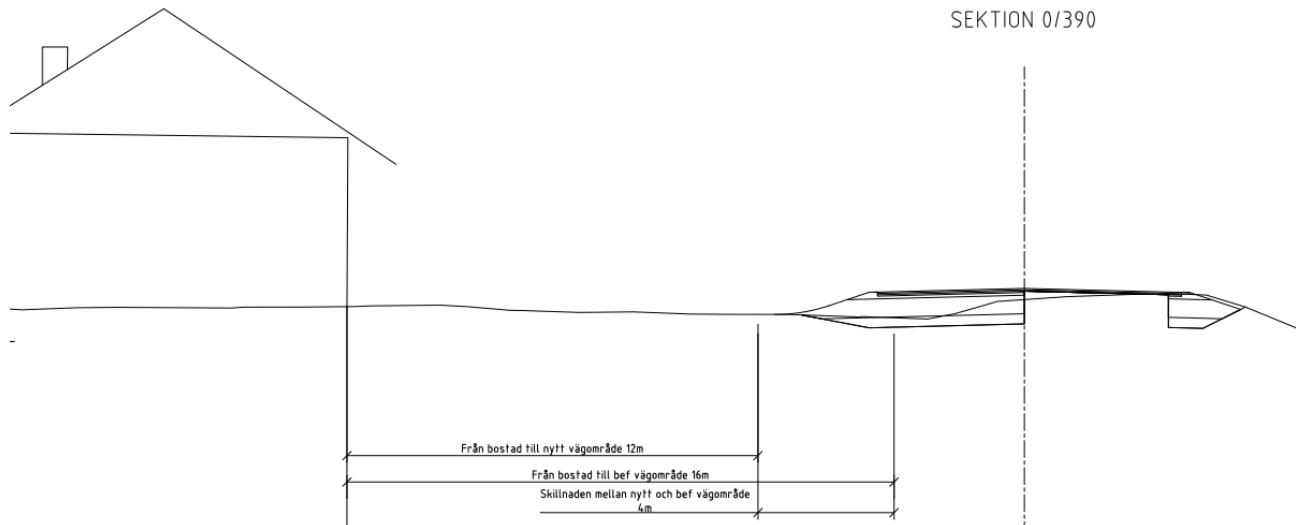
Figur 14. Sektion över intrång på en fastighet av alternativ korsningsåtgärder.
