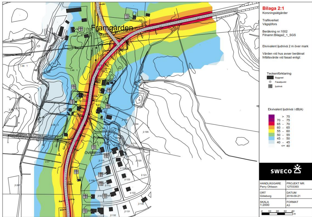
Figur 16. Bullerberäkning av ekvivalent ljudnivå i alternativ korsningsåtgärder.
