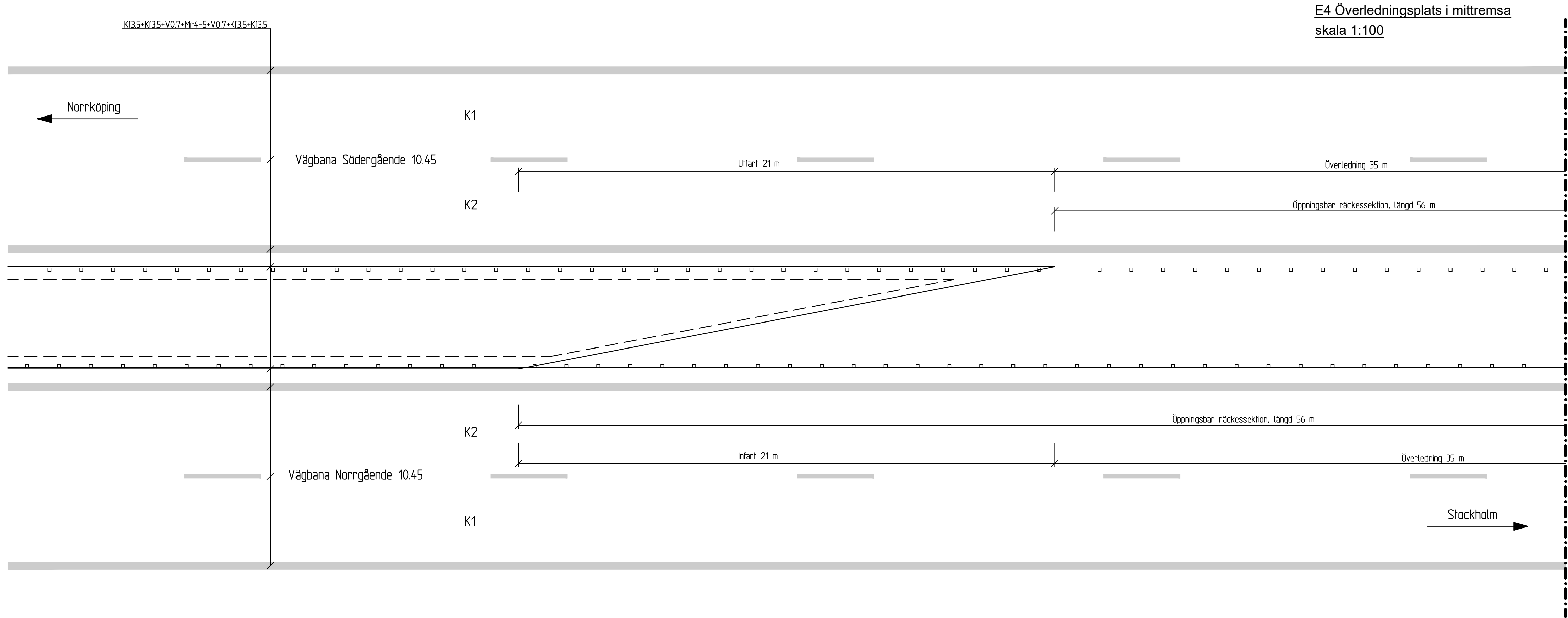
E4 Överledningsplats i mittremsa skala 1:100
