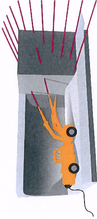
Borrning för injektering
