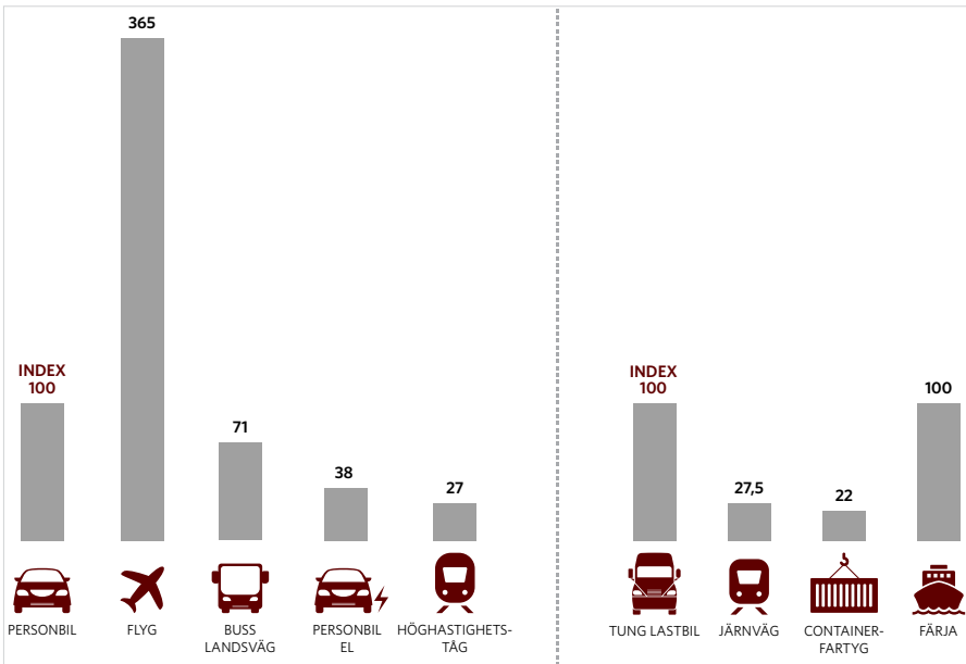
Figur 5.13 Värden för persontransporter (vänster) är jämförda mot energianvändning (kWh/pkm) för personbil på landsväg = index 100. Värden för godstransporter (höger) är jämförda mot energianvändning för tung lastbil, fjärrtransport = index 100 (Trafikverket, 2021i).
