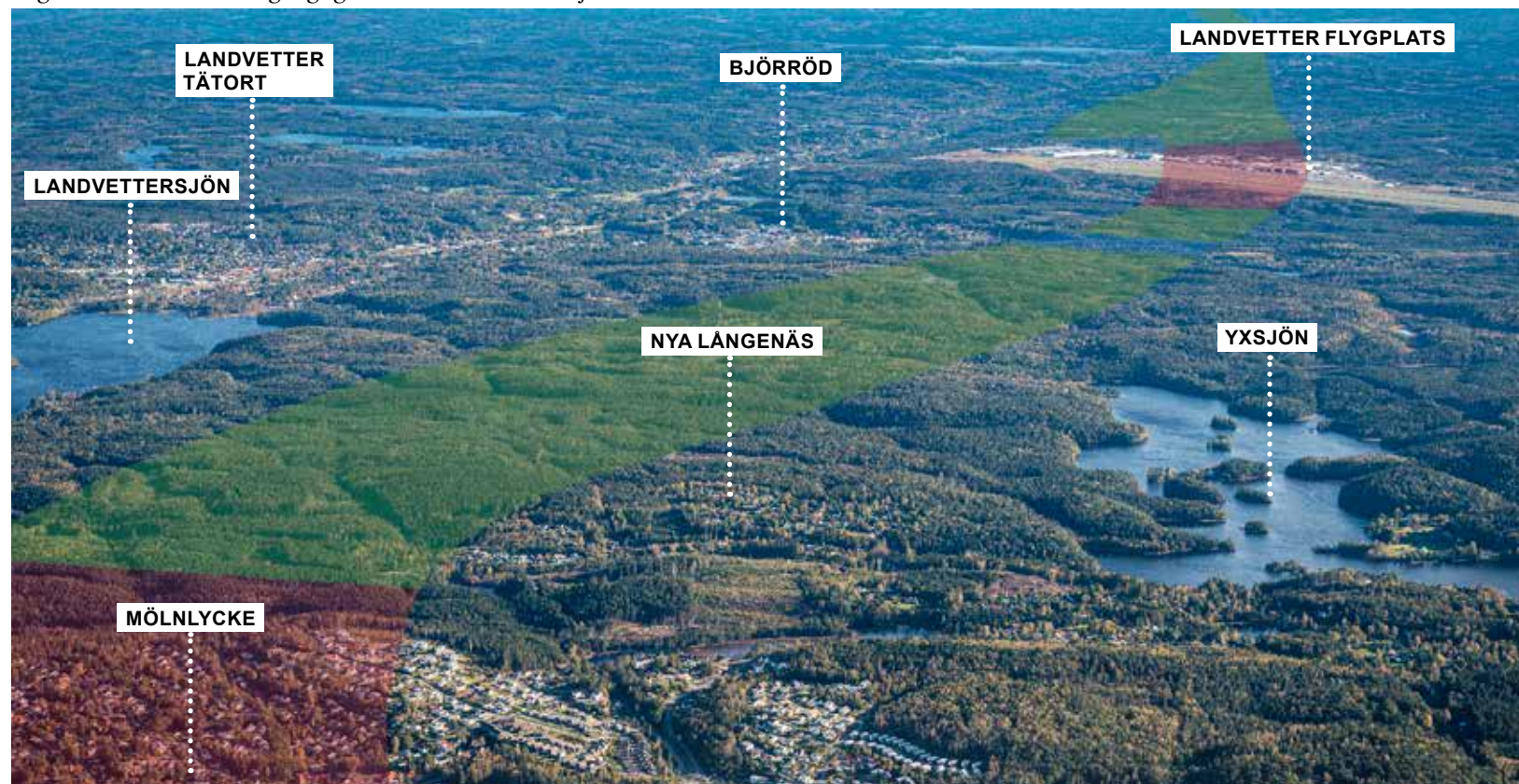
Figur 81. Flygfoto över Yxsjöns naturreservat med korridoralternativ illustrerat i bild, vy mot öster. Den röda färgen illustrerar bergtunnel och den gröna färgen illustrerar anläggning i markplan. Till vänster syns Landvettersjön och till höger syns Yxsjön. Närmast i bild syns östra delarna av Mölnlycke och längre bort i bild syns Landvetter flygplats. (Foto: Per Pixel, 2020)
