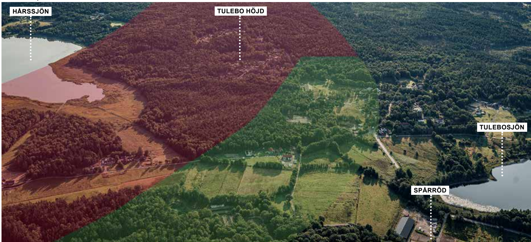
Figur 79. Flygfoto över fokusområdet Tulebo med korridoralternativ illustrerat i bild, vy mot öster. Den röda färgen illustrerar bergtunnel och den gröna färgen illustrerar anläggning i markplan. I bilden syns Hårssjön till vänster och Tulebosjön till höger. Mellan sjöarna finns jordbrukslandskap och bostadsbebyggelse. (Foto: Per Pixel, 2020)
