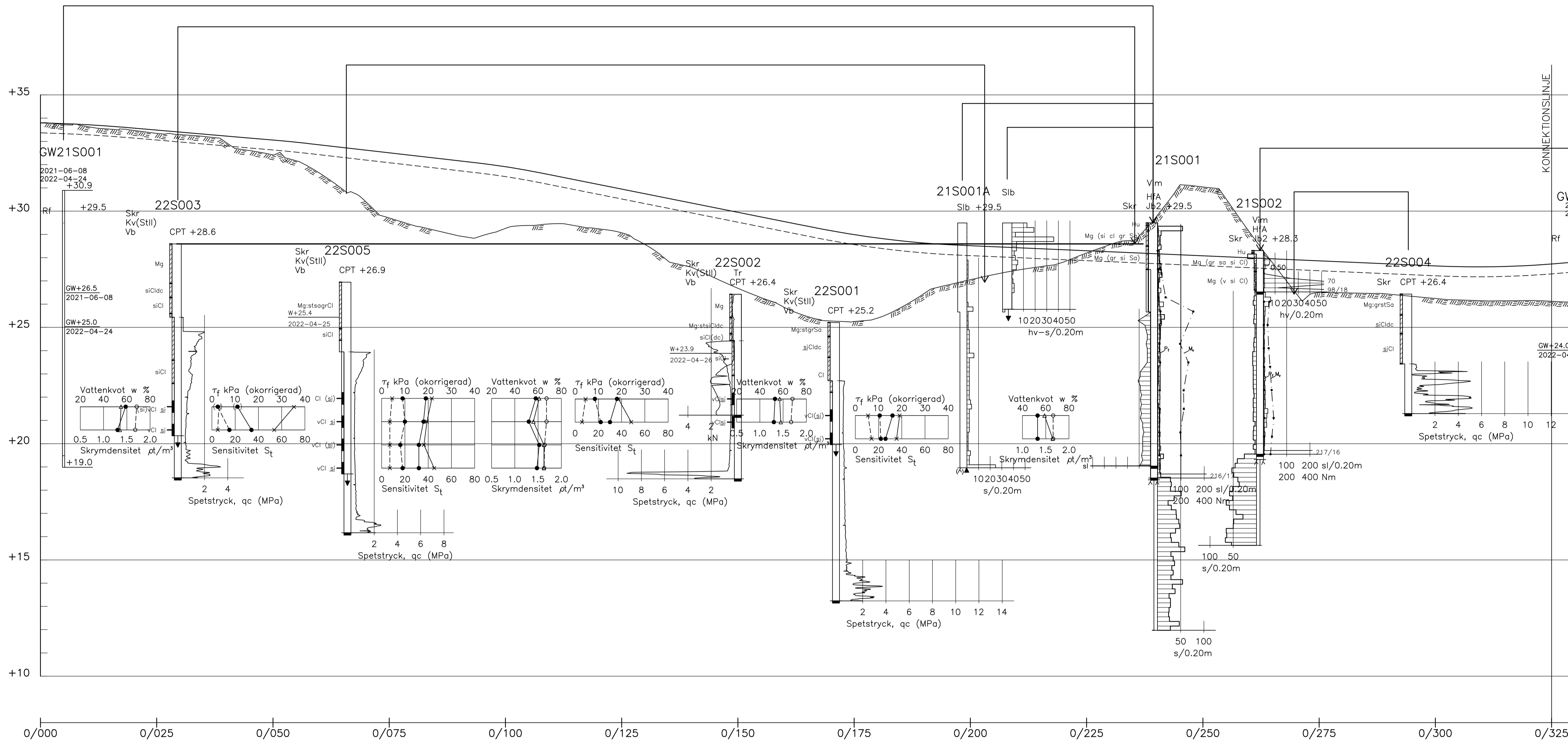
PROFIL GC-VÄG H 1: 100 L 1: 500
