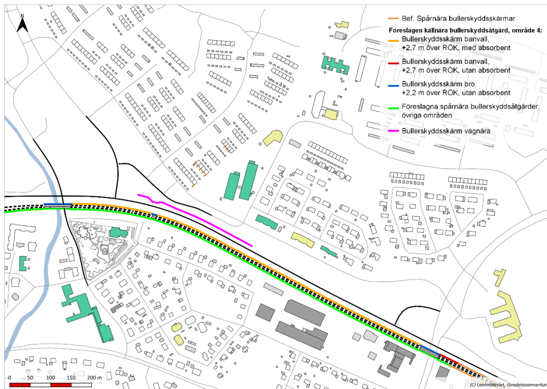
Figur 6.10. Översiktfigur för föreslagna källnära bullerskyddsåtgärder för område 4 – Sjungande dalen.
