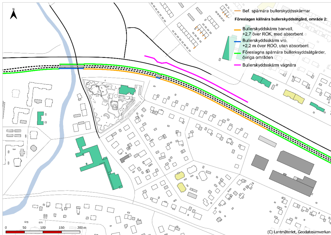
Figur 6.6. Översiktfigur för föreslagna källnära bullerskyddsåtgärder för område 2 – Brännan.
