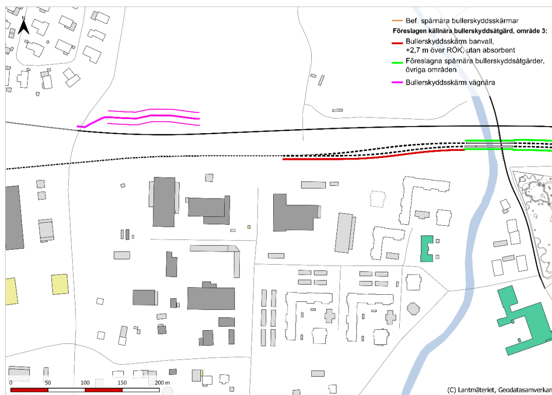
Figur 6.8. Översiktfigur för föreslagna källnära bullerskyddsåtgärder för område 3 – Degerbyn.
