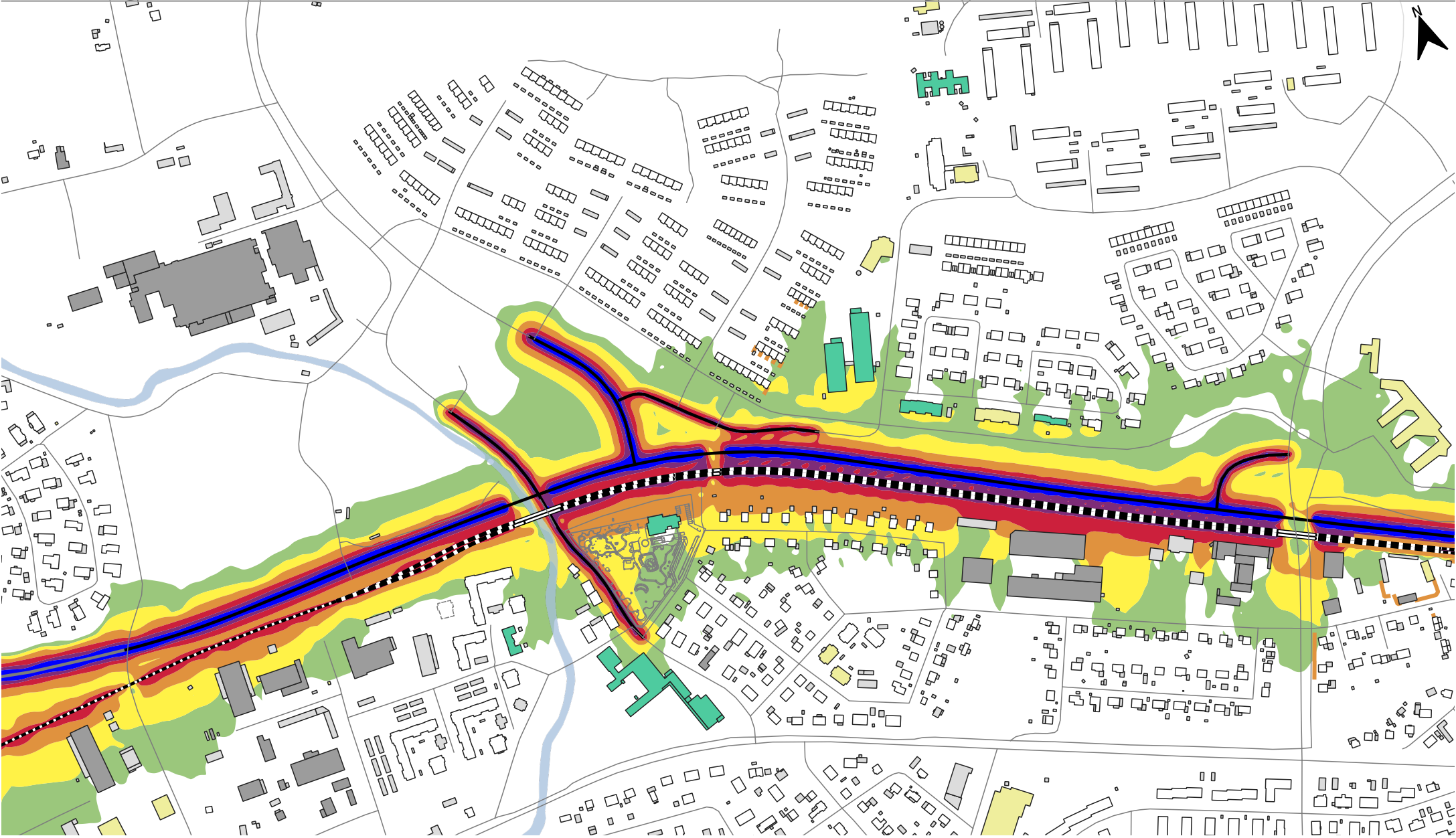
Planförslaget 2040 utan föreslagna källnära bullerskyddsåtgärder - Maximal ljudnivå, Lmax,dag, för all statlig och ombyggd infrastruktur
