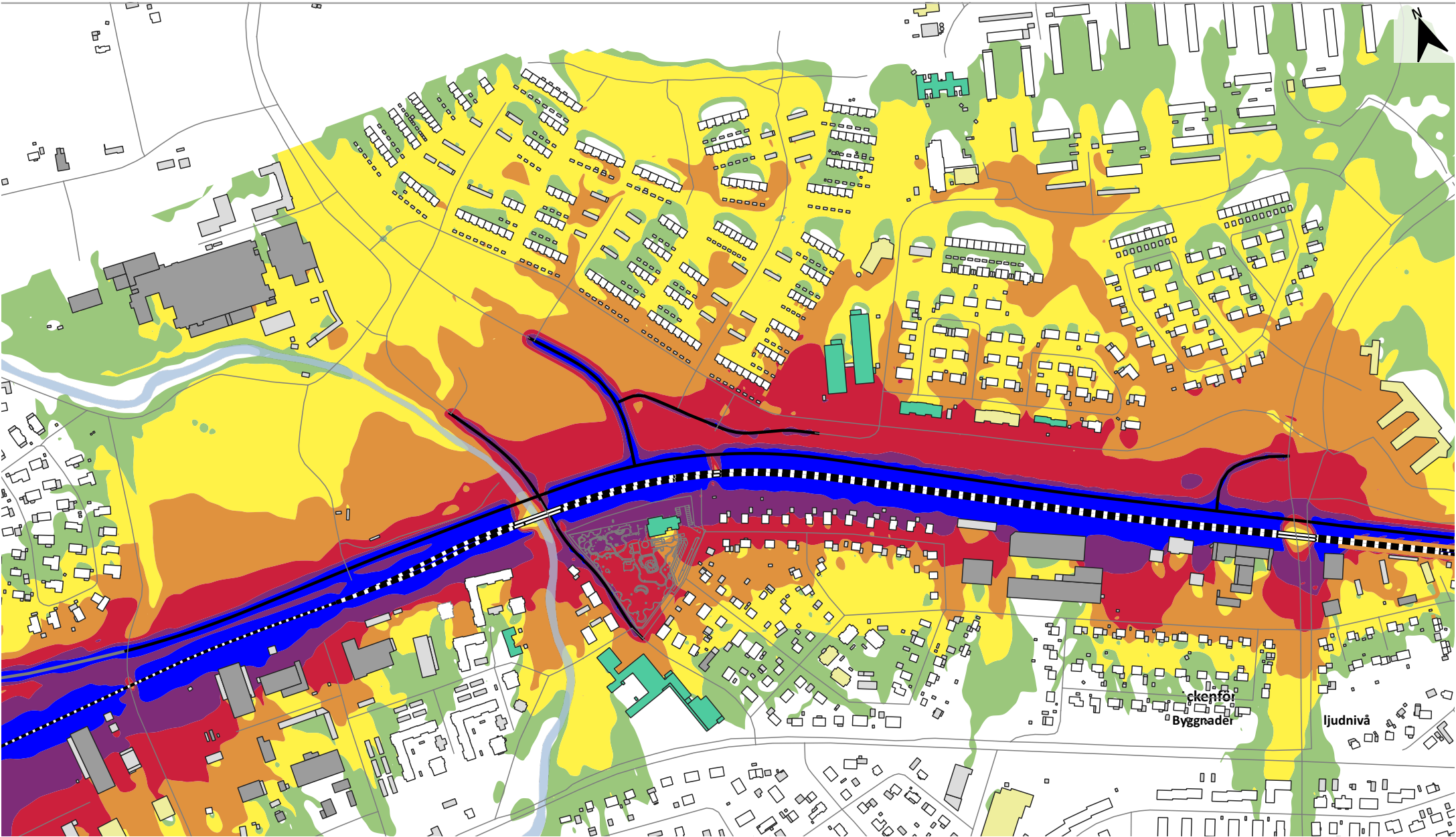
Planförslaget 2040 utan föreslagna källnära bullerskyddsåtgärder - Maximal ljudnivå, Lmax,natt, för all statlig och ombyggd infrastruktur
