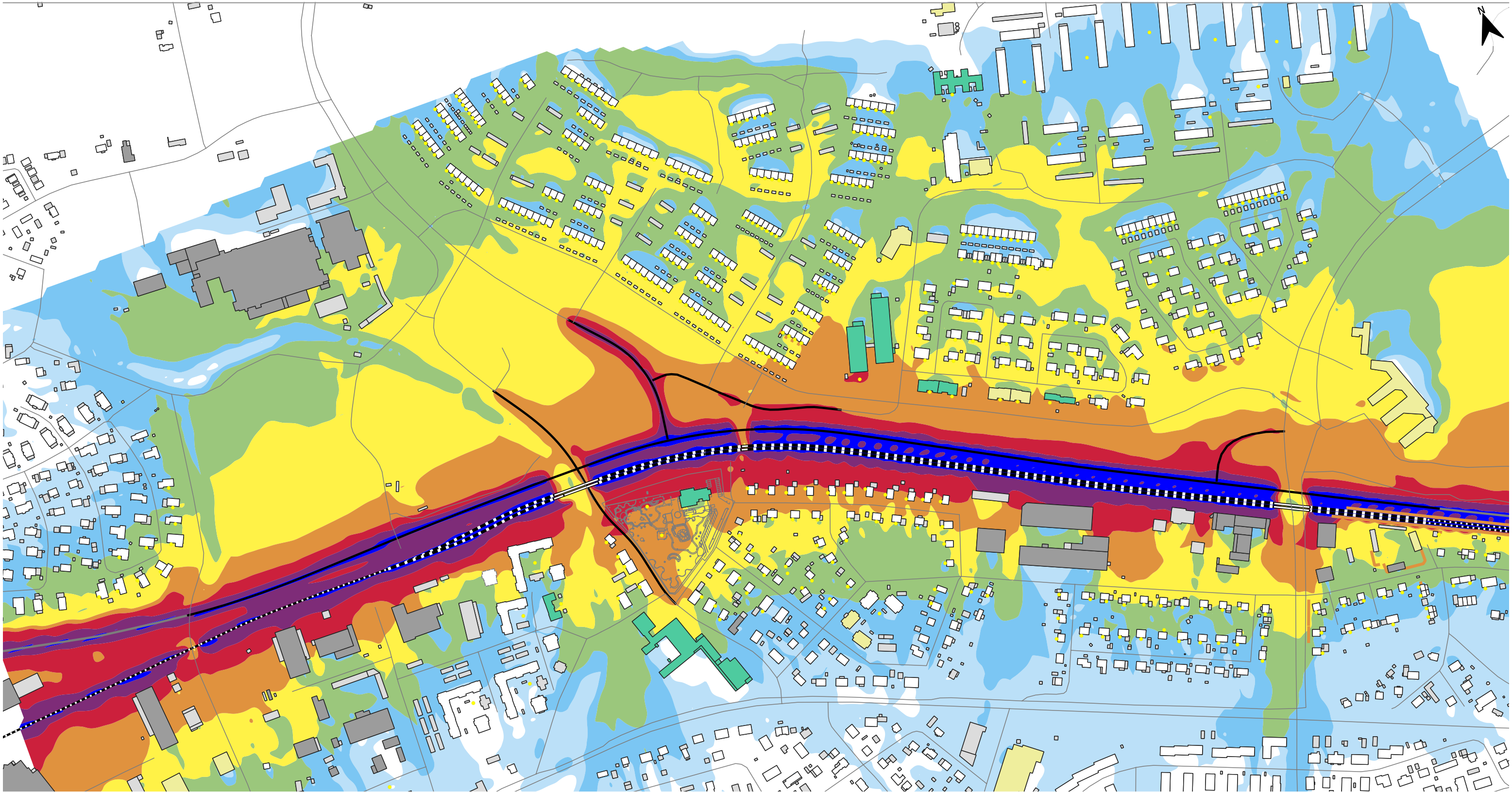
Planförslaget 2040 utan föreslagna källnära bullerskyddsåtgärder - Ekvivalent ljudnivå, Leq, för all statlig och ombyggd infrastruktur
