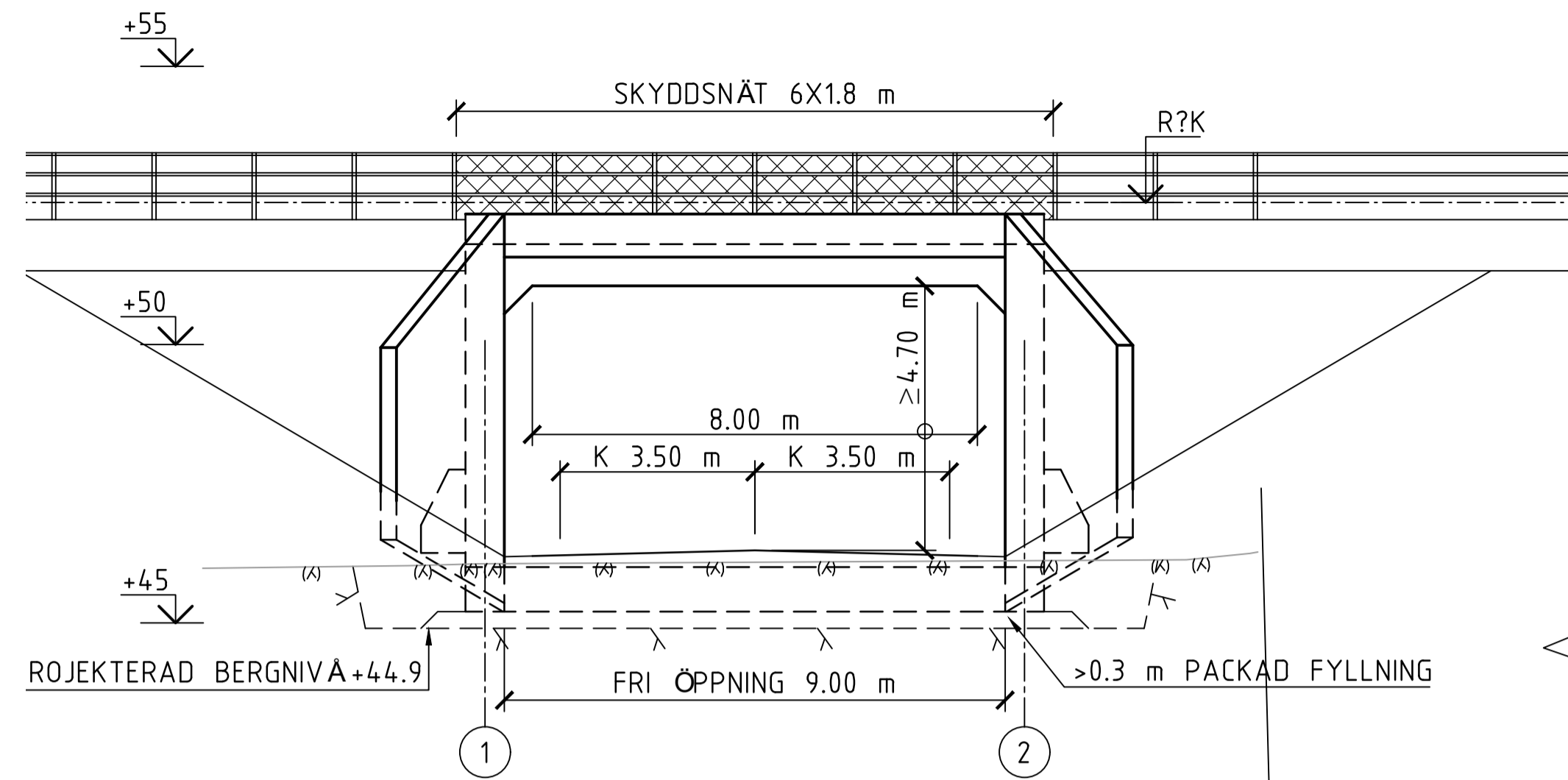
ELEVATION A-A 1:100
