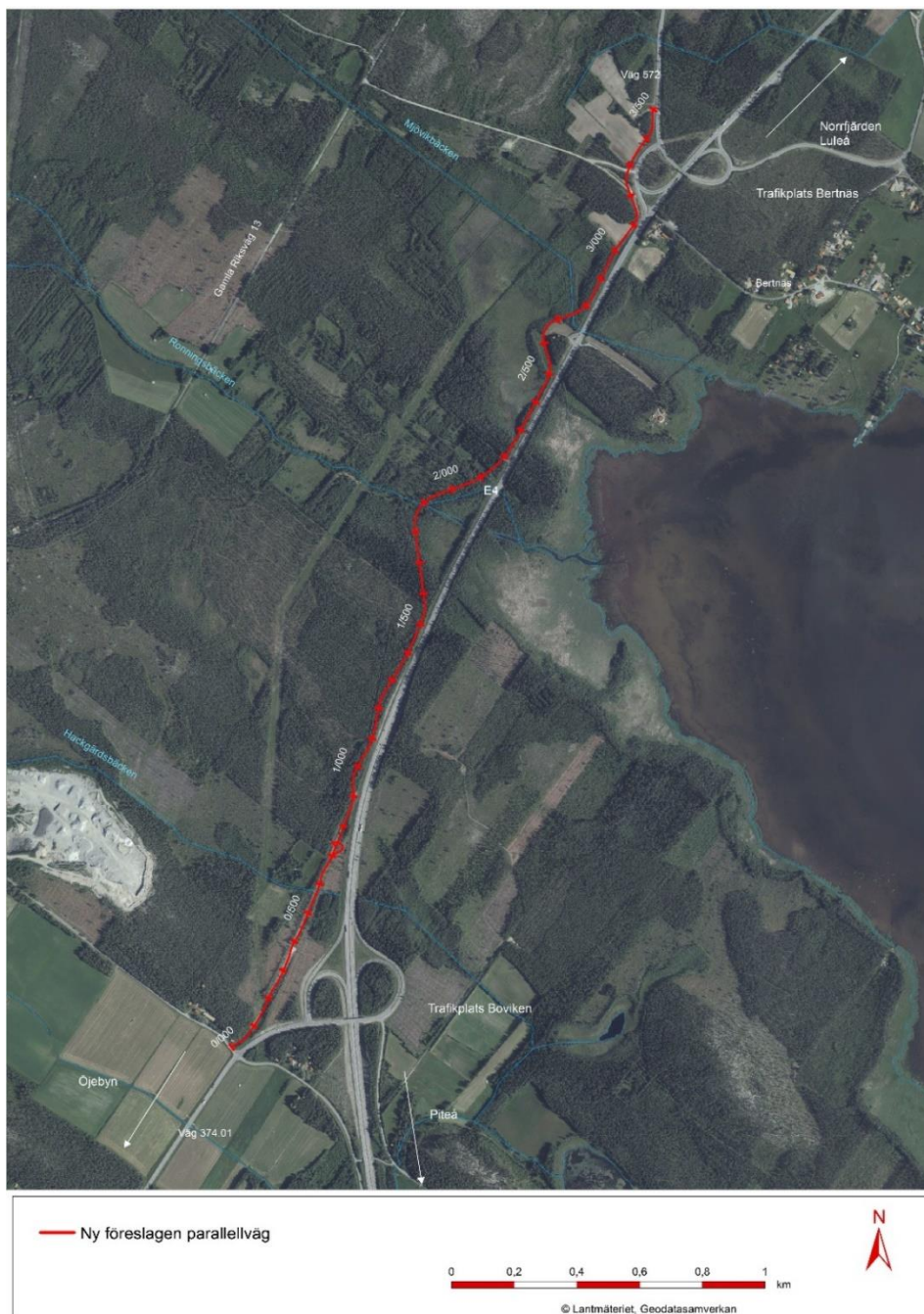
Figur 5.2-1. Sträckning av föreslagen parallellväg med längdmätning.
