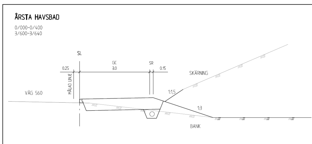
Figur 13. Gång- och cykelbana med kantstöd dikt mot befintlig väg. Teckenförklaring: GC = gång- och cykelväg, SR = stödremsa och SL = stakad linje
