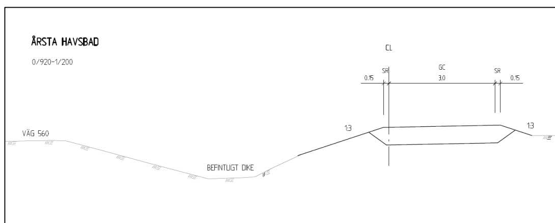
Figur 15. Gång- och cykelväg med skiljeremsa vid låg bank och dike.
