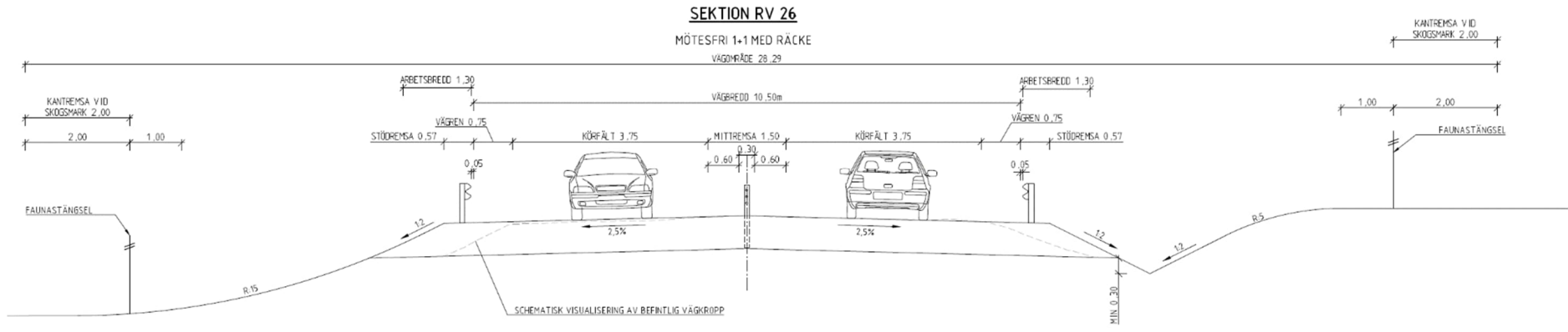
Figur 12. Sektion väg 26. Mötesfri 1+1 med räcke, se ritning 100T0401.
