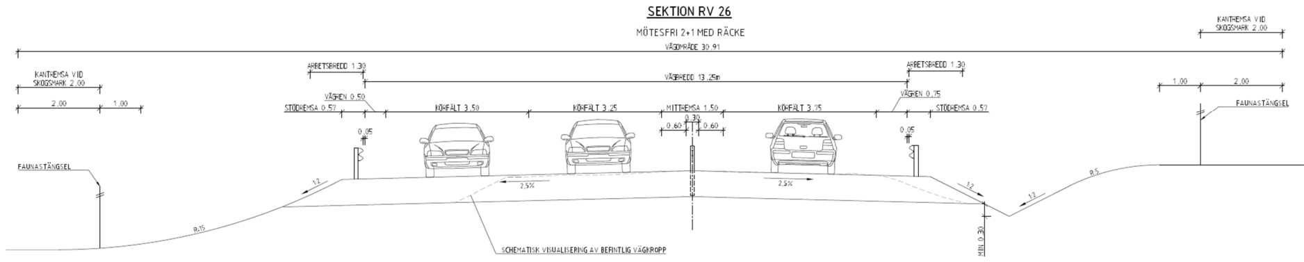
Figur 13. Sektion väg 26. Mötesfri 2+1 med räcke, se ritning 100T0402.
