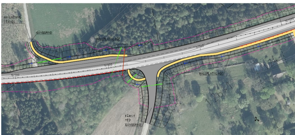
Figur 15. Korsningen vid längdmätning 9/850 utformas med ett separat körfält för vänstersvängande.
