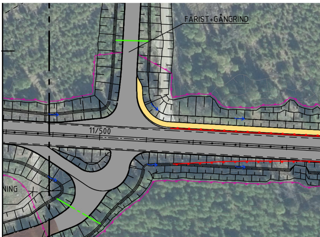
Figur 14. Korsningen vid längdmätning 11/530 utformas med ögla.
