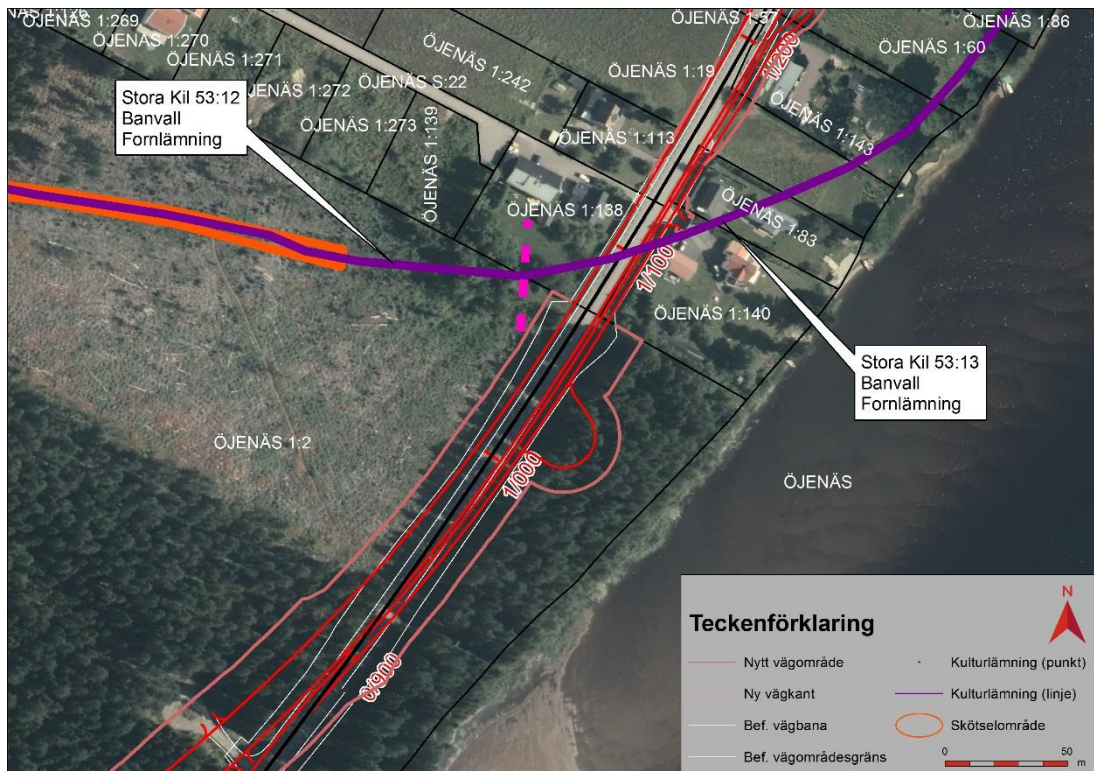
Figur 24. Planerade åtgärder intill fornlämningsklassad banvall.
