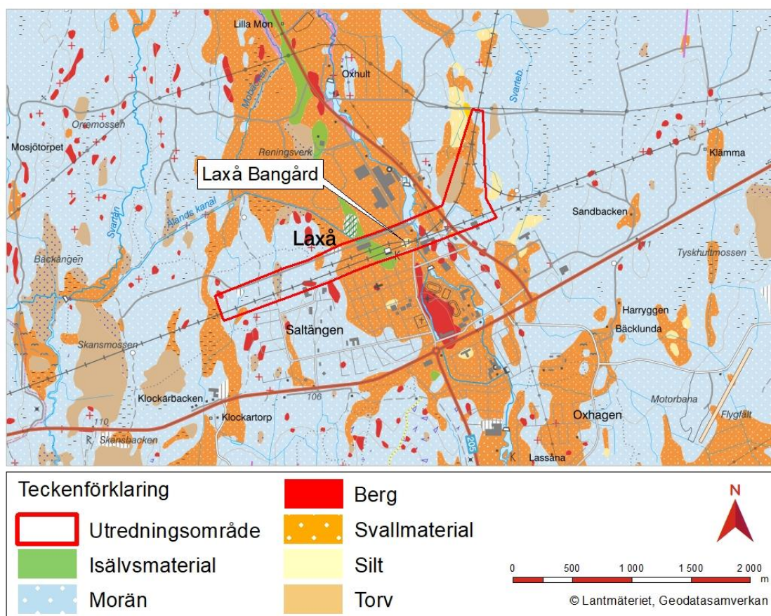
Figur 17. Jordartskarta över närområdet och utredningsområdet till Laxå Bangård.
