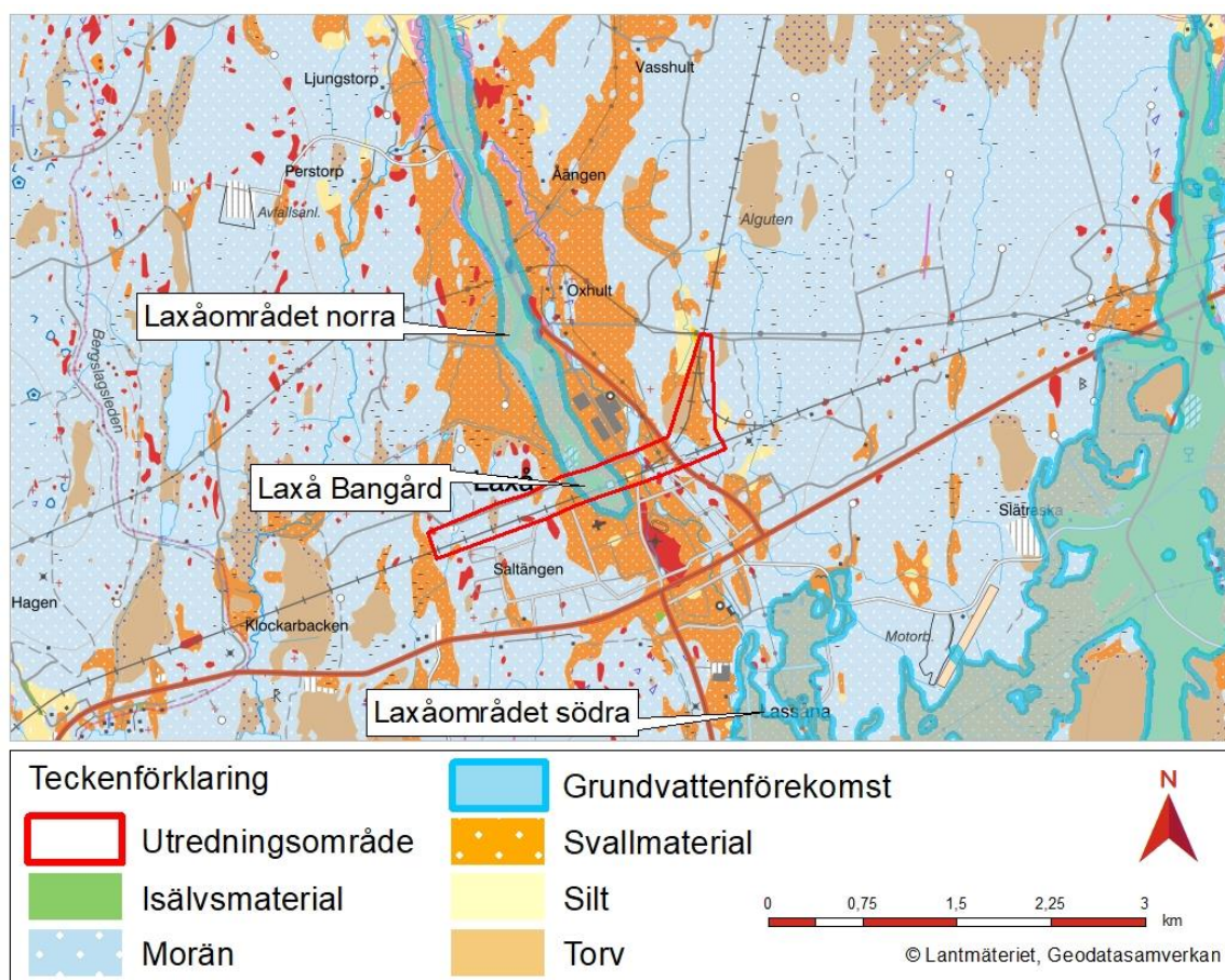
Figur 18. Jordartskarta med grundvattenförekomster i närområdet till Laxå Bangård.
