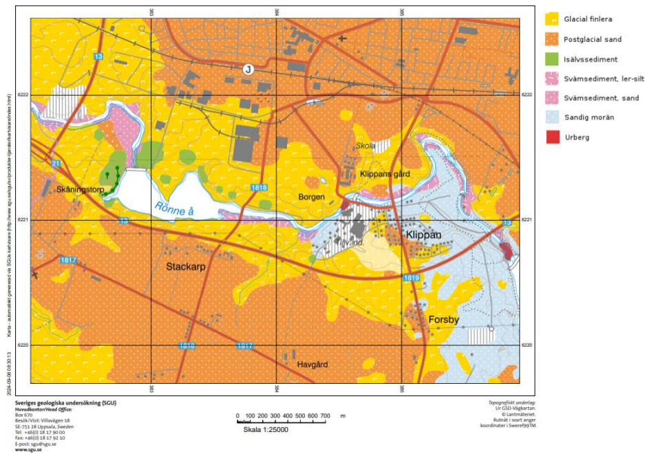
Figur 35 Jordartskarta från västra delen av vägsträckan, från trafikplats Skåningstorp till där Rönne å korsar väg 21.
