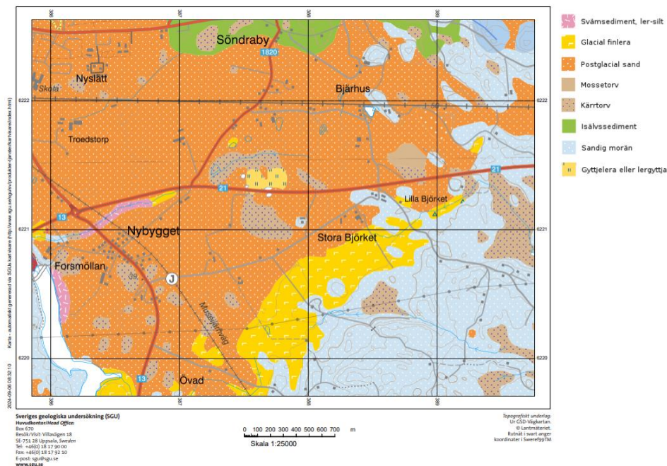
Figur 36 Jordartskarta från mellersta delen av vägsträckan, från Forsmöllan till Lilla Björket.
