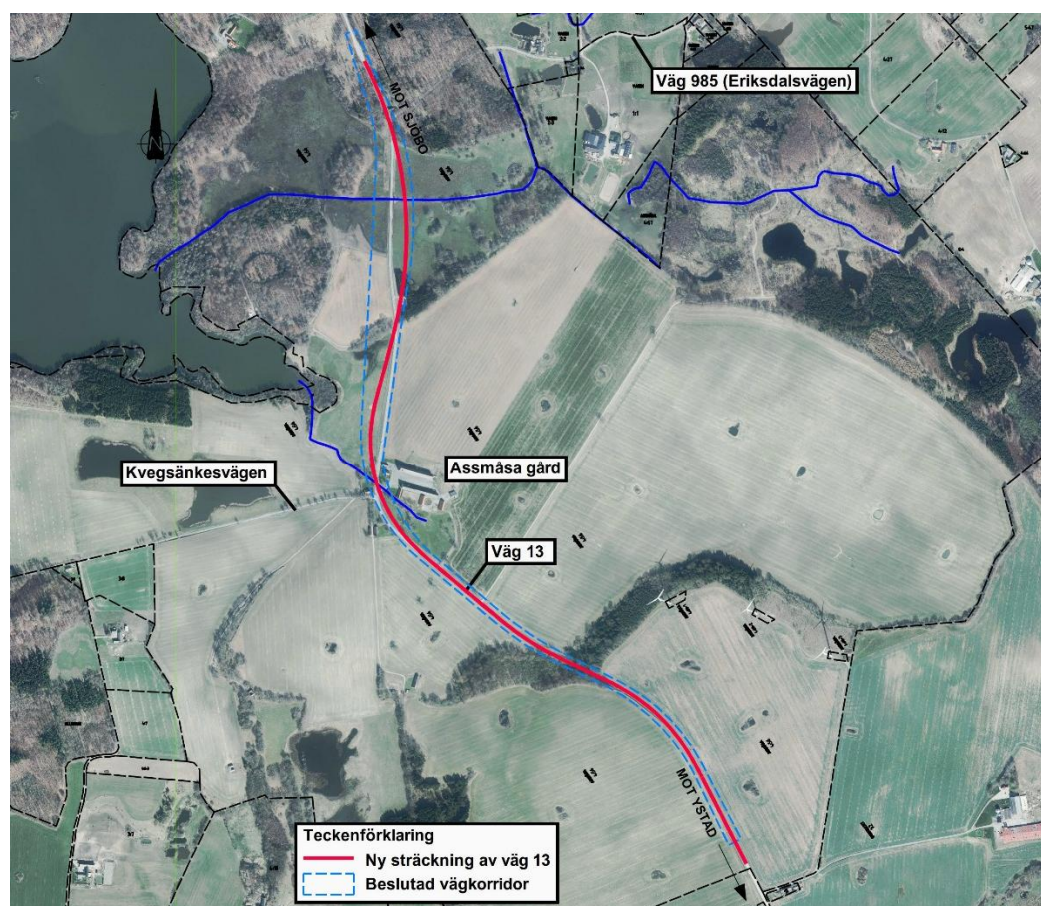
Figur 4.2.1: Föreslagen väglinje inom beslutad vägkorridor
