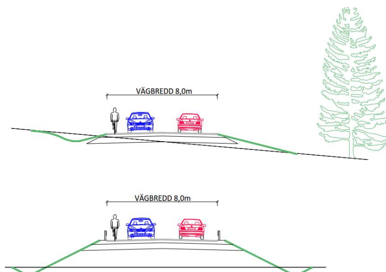
Figur 4.2.2:1 Vägsektion i skärning och bank för väg 13
