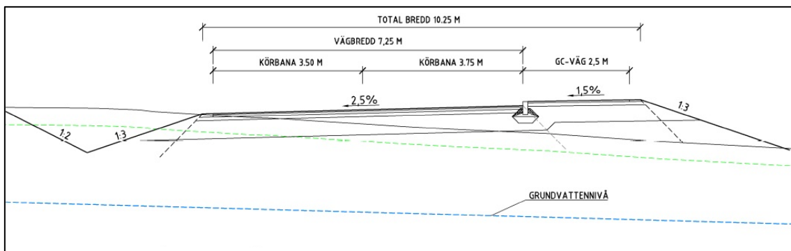
Typsektion B
