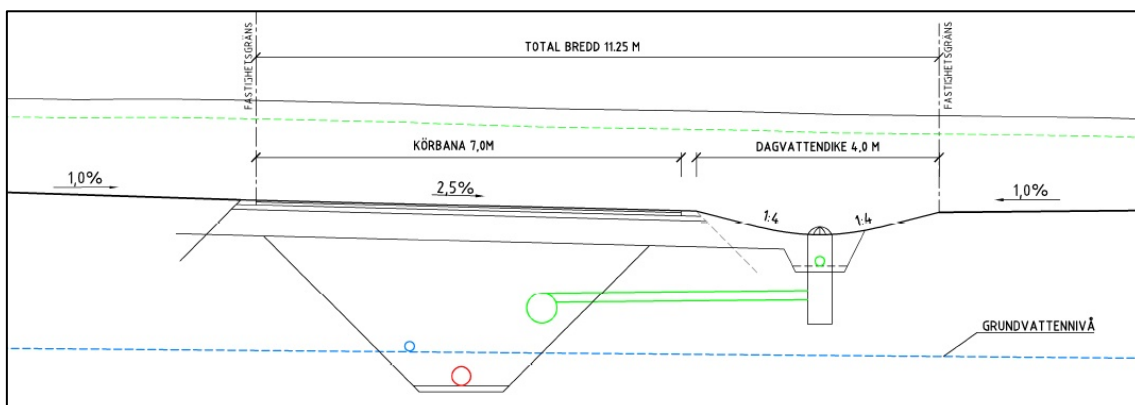
Typsektion D
