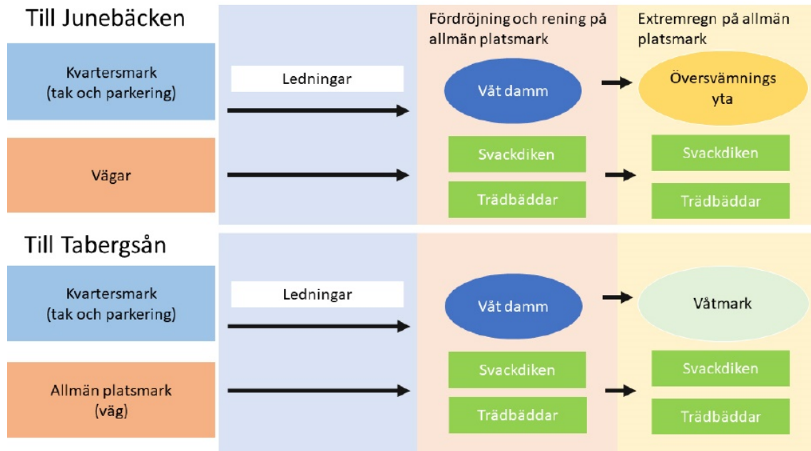
Flödesschema för dagvattenhanteringen inom planområdet. Från dagvattenutredningen
