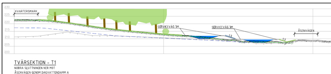
Marksektion T1 vid Åsens gård. Från vänster syns den befintliga lövträdslänten, två dagvattendammar samt Åsensvägen.
