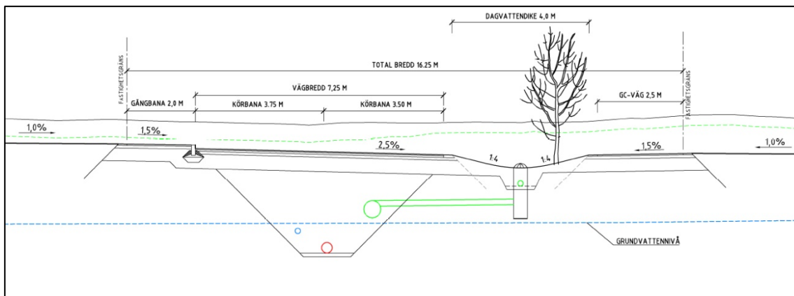
Typsektion A
