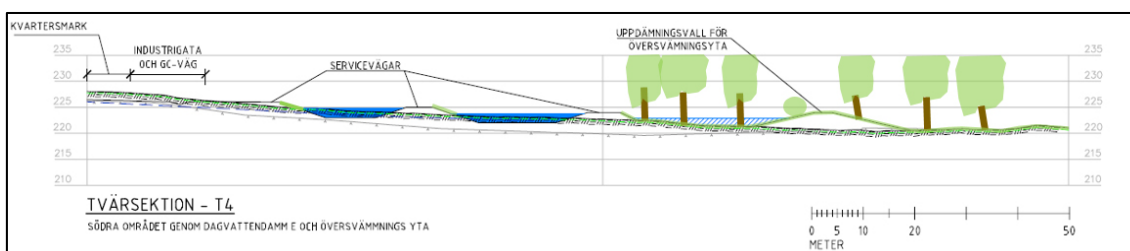
Marksektion T4 genom planerad översilningsyta och fördröjningsdammar.
