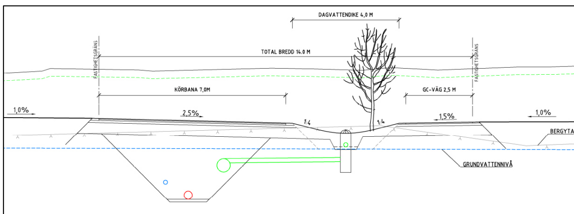
Typsektion C (förekommer även utan trädplantering)
