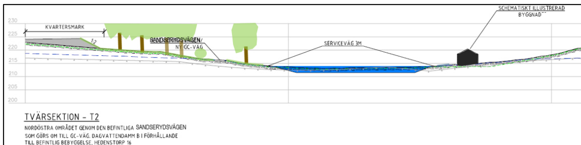
Marksektion T2 vid befintlig bebyggelse vid Dylycke. Från vänster syns den befintliga lövträdslänten, Sandserydsvägen ombyggd till cykelväg, ny dagvattendamm samt det närmaste bostadshuset.
