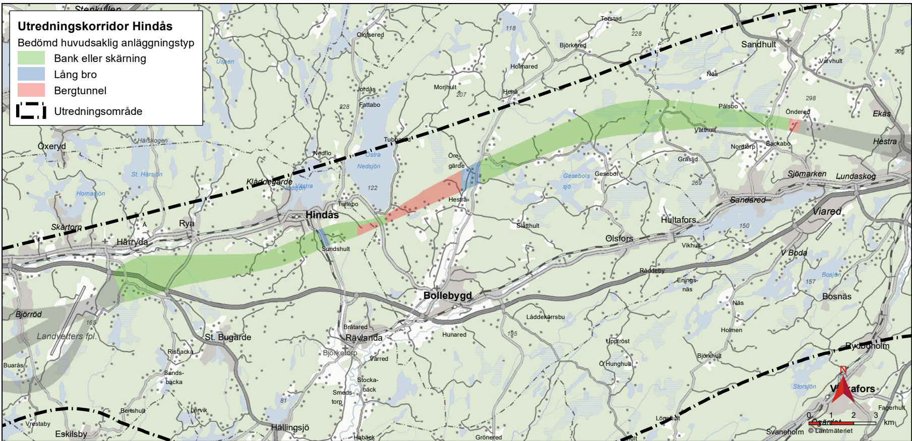
Figur 206. Utredningskorridor Hindås.
