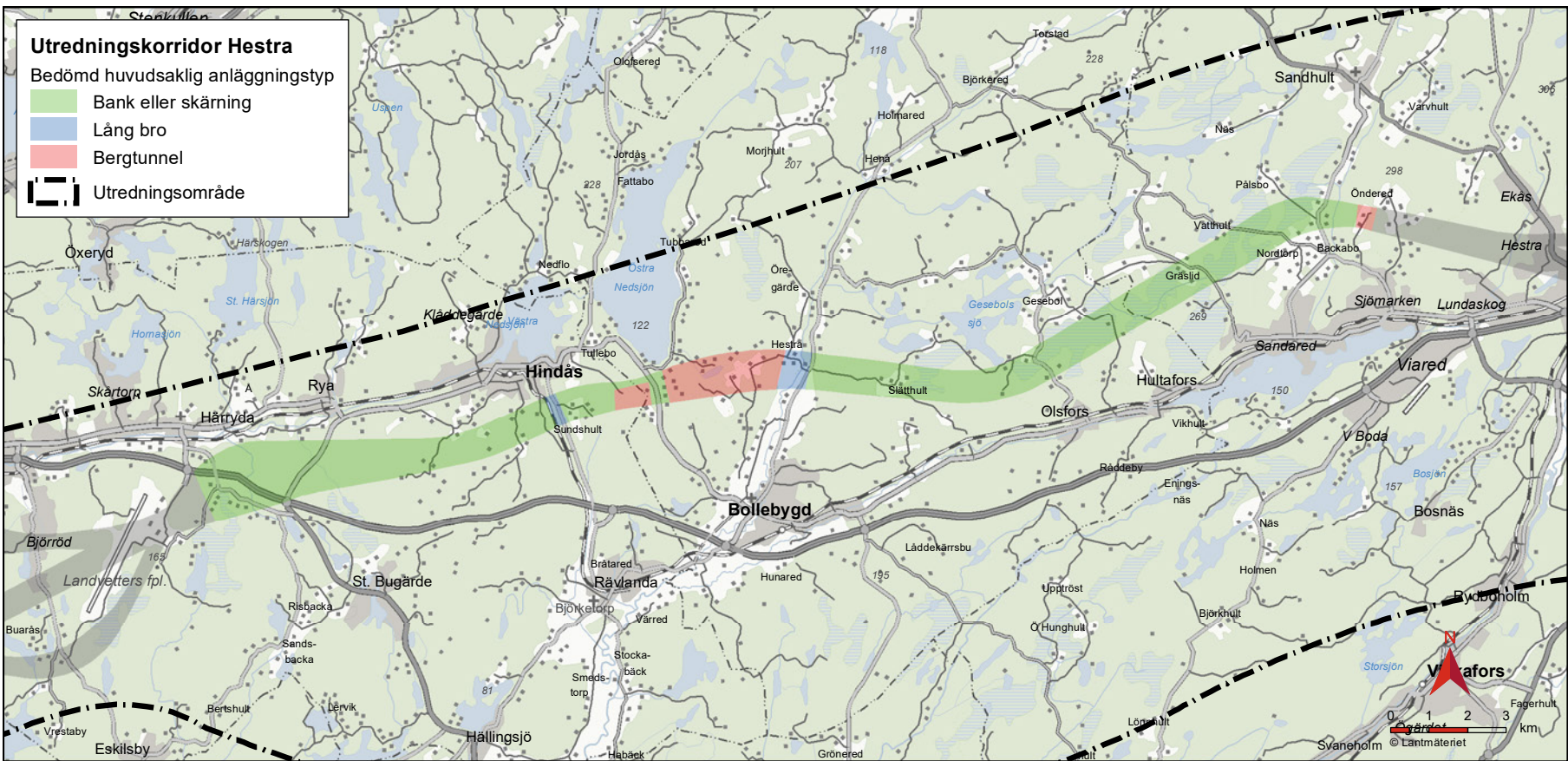
Figur 207. Utredningskorridor Hestra.
