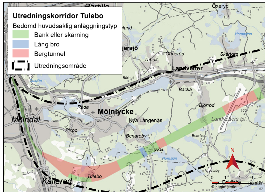
Figur 203. Utredningskorridor Tulebo.
