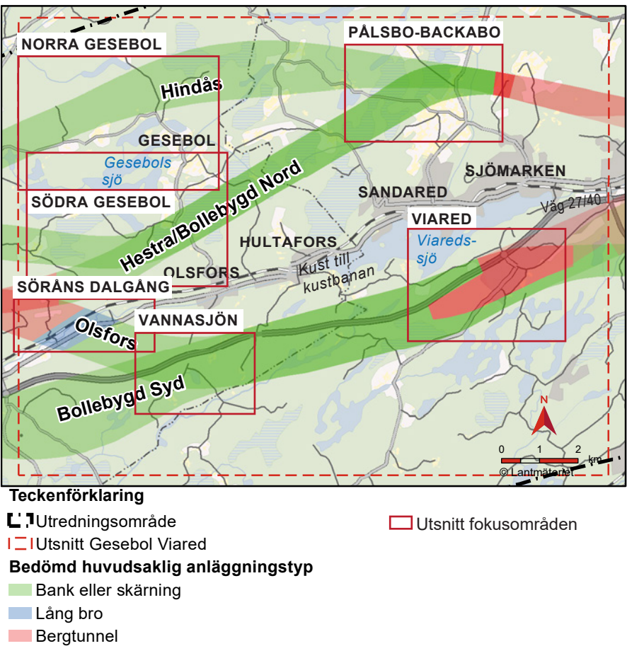
Figur 147. Översiktsskarta med anläggningstyper, korridorer och fokusområden vid Gesebol och Viared.
