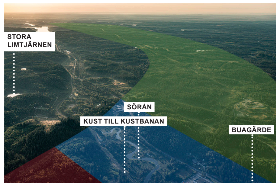
Figur 155. Flygfoto över Söråns dalgång med korridorsalternativ illustrerat i bild, vy mot sydost. Den röda färgen illustrerar bergtunnel, den blå färgen illustrerar bro och den gröna färgen illustrerar anläggning i markplan. (Foto: Per Pixel, 2020)
