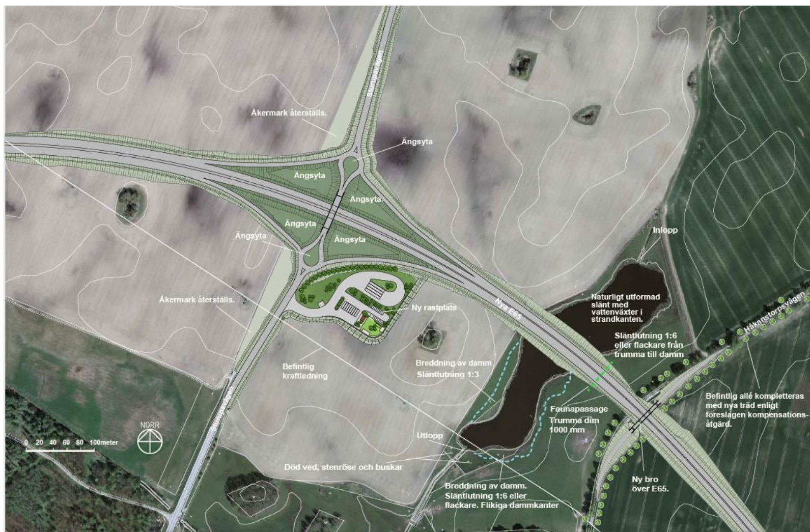
Figur 17. Utformning av ny trafikplats vid väg 813 (Sturupsvägen), ny rastplats, damm i öster samt Håkanstorpsallén med föreslagna kompensationsåtgärder.
