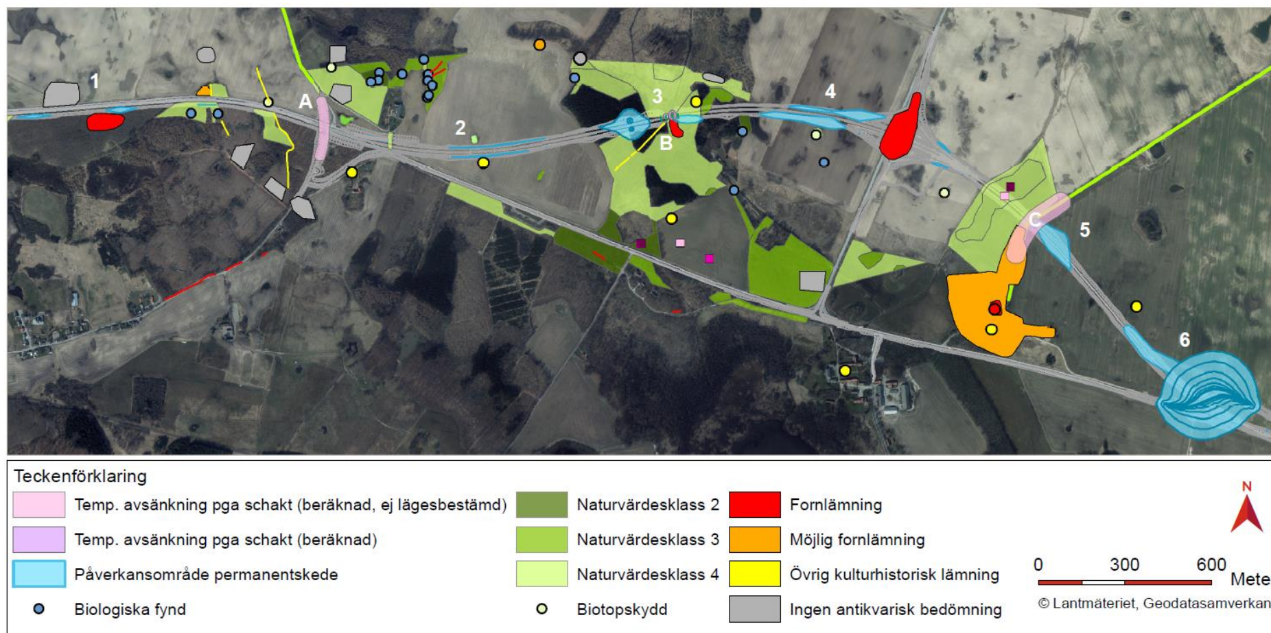
Figur 97. Översikt av vägsträckan med förväntade grundvattenavsänkningar i bygg- och driftskede i förhållande till skyddsobjekt, om inga åtgärder vidtas. Observera att vissa temporära avsänkningar under schaktarbete (rosa polygoner) är ungefärligt utritade då schaktens exakta läge ej är fastställt.
