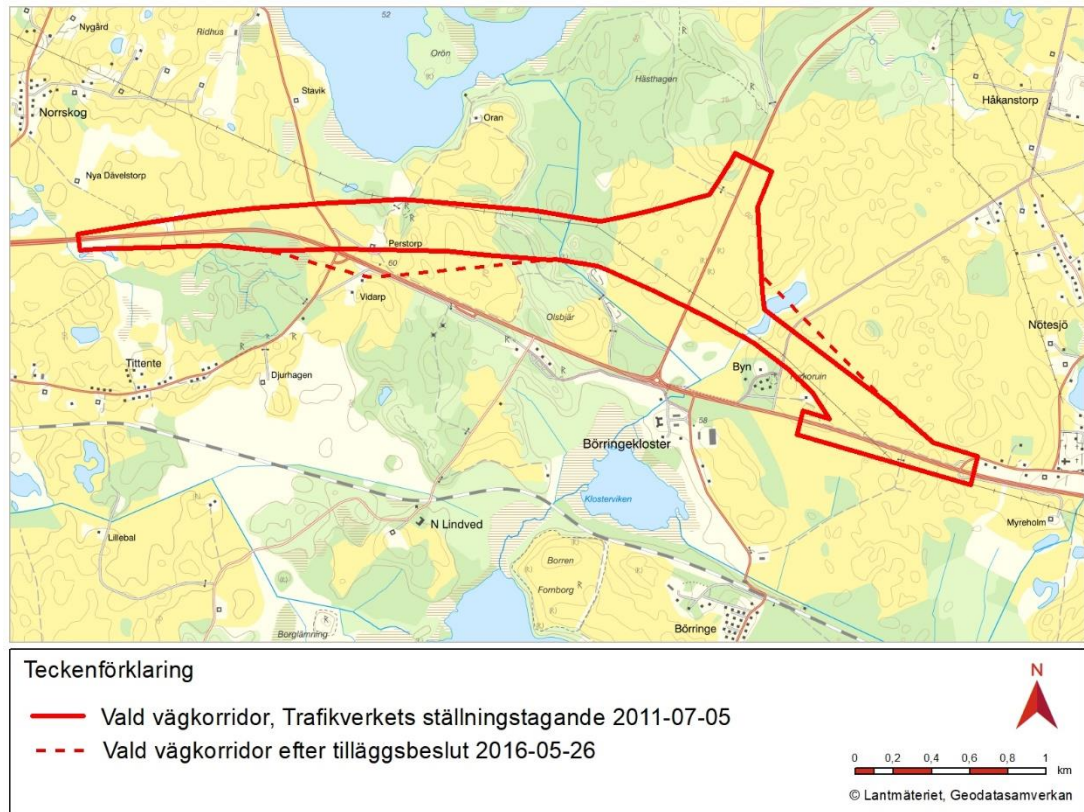
Figur 26. Vald vägkorridor Norr efter tilläggsbeslut 2016-05-26 Bild: Tolkning av AFRY.
