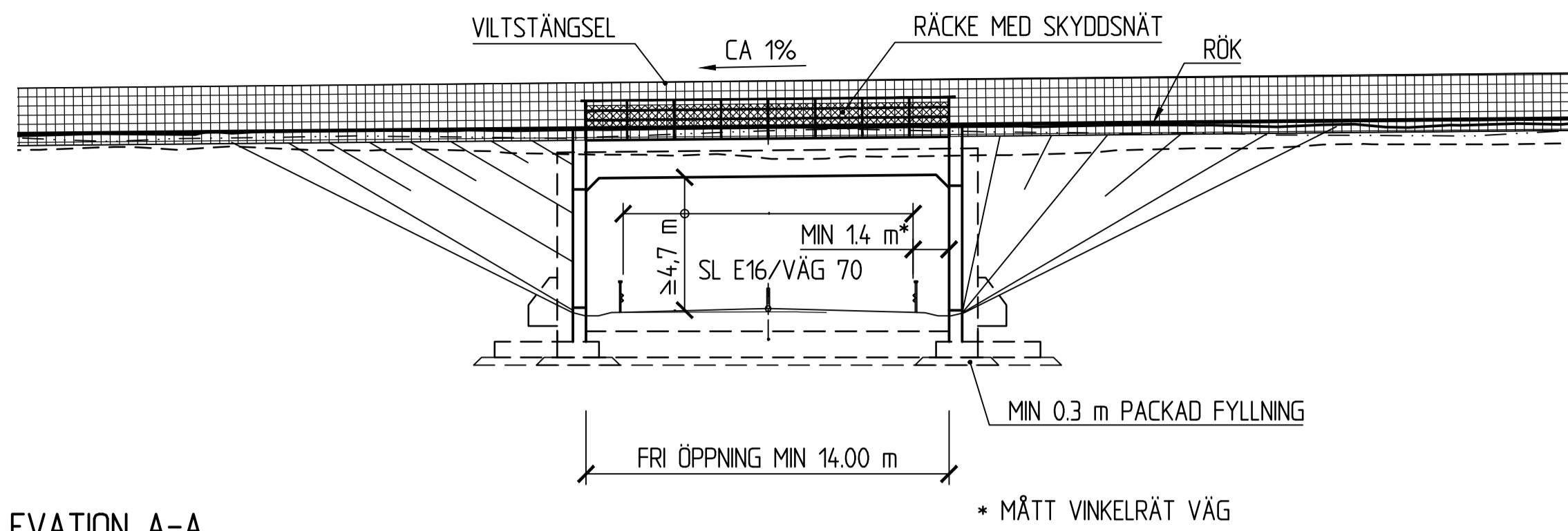
ELEVATION A-A 1:200
