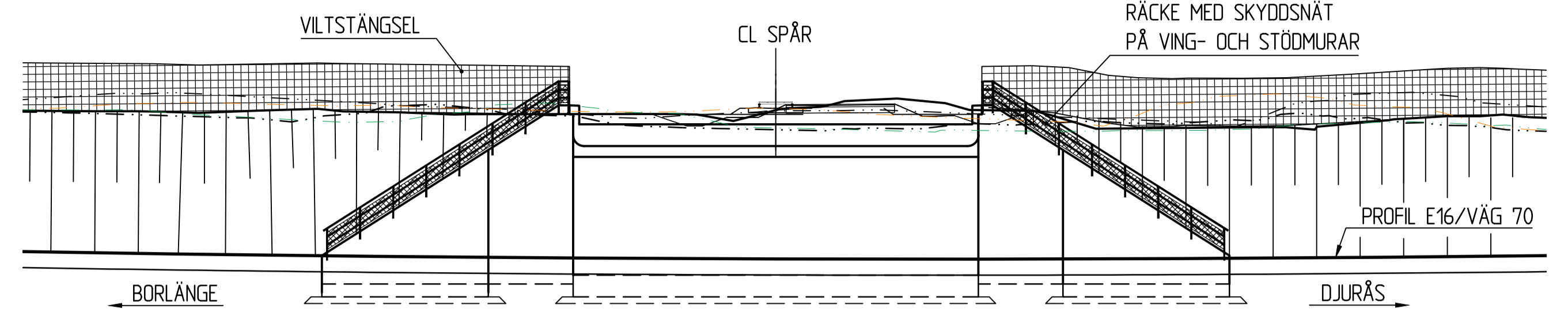
SEKTION B-B 1:200
