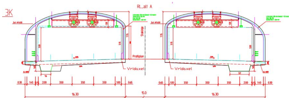
Figur 3-2. Typsektion huvudtunnlar med 3-körfält.
