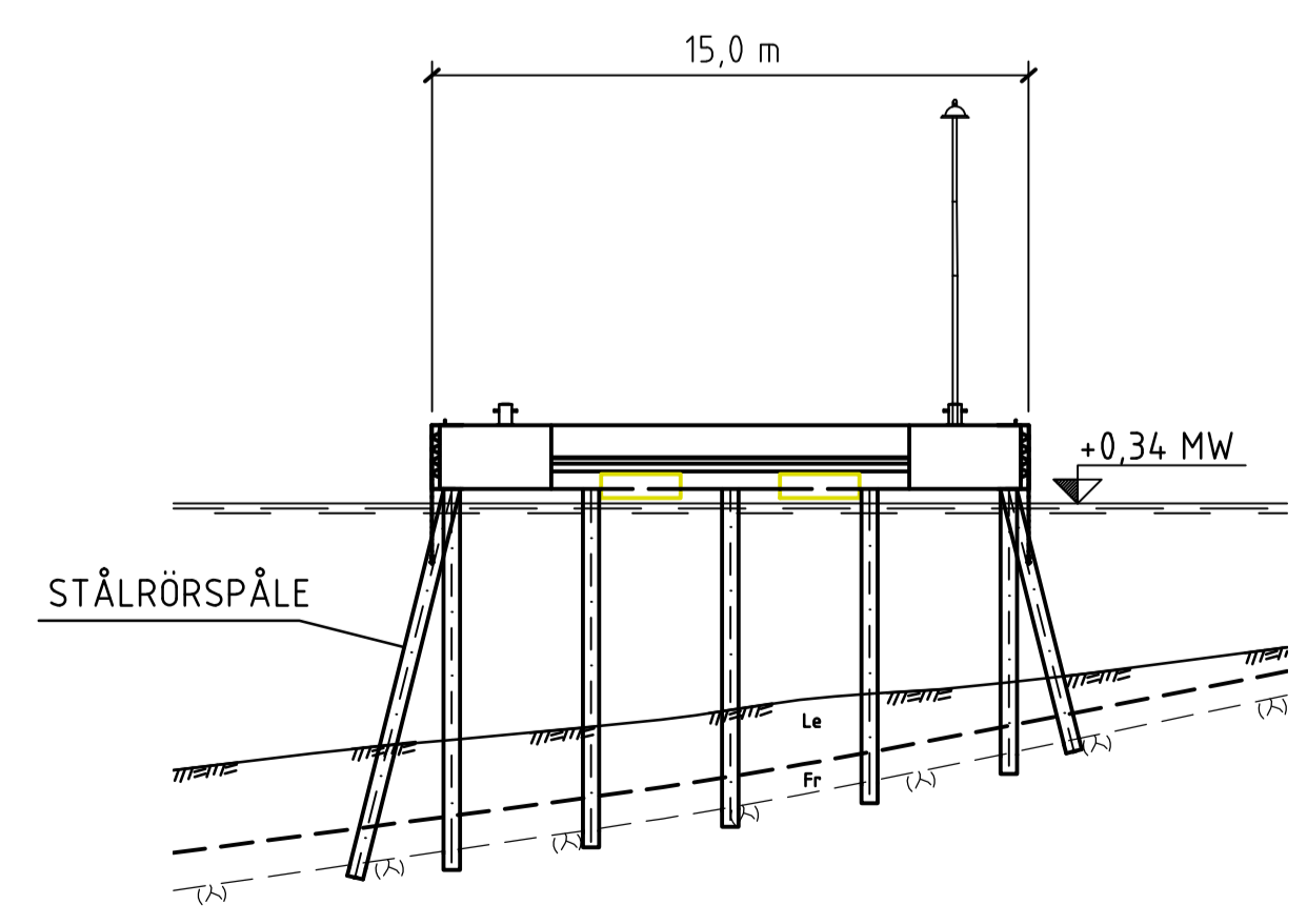
ELEVATION B-B 1:200
