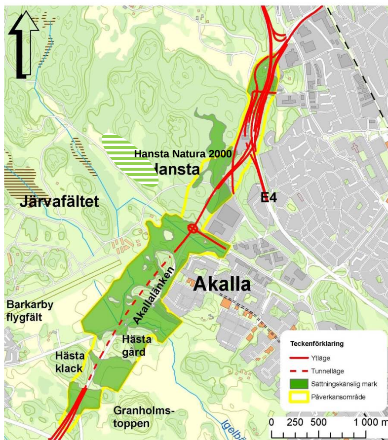
Figur 4.2 Påverkansområde med åtgärder enligt av Trafikverket till domstolen föreslagna villkor för grundvattenbortledning (illustration ur MKB till ansökan), bilden kompletterad med Natura 2000-området inlagt som symbol, för exakta gränser se figur 3.1.
