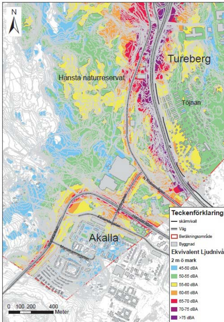
Figur 11. Bullerberäkningar nollalternativ
