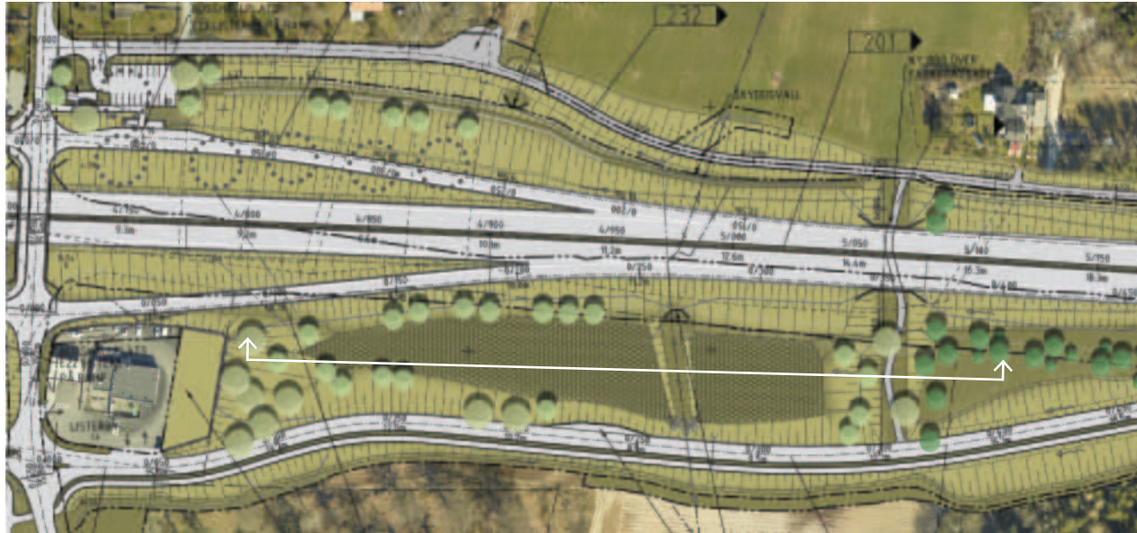
Figur 28. Illustration av Listerby trafikplats, öster om bron: Dagvattendammar och faunapassage. Öster om bron förläggs ny E22 norr om befintlig väg. Lokalväg och cykelväg går i kanten av befintlig ekdunge och leds österut mot Förkärla i samma läge som befintlig väg. Ersättningsvägar, av- och påfarter till den nya bron, lokalväg och ny motorväg har anpassats till landskapet men har ändå medfört att fler hus behöver rivas. En hög bullervall och dagvattenmagasinen blir nya inslag i landskapet. Nya träd har illustrerats vid pendlarparkeringar, dammar och faunapassage samt där befintlig E22 rivs och återställs med skog. (Prickad cirkel representerar fastighet som löses in) Sektion enligt figur 29.
