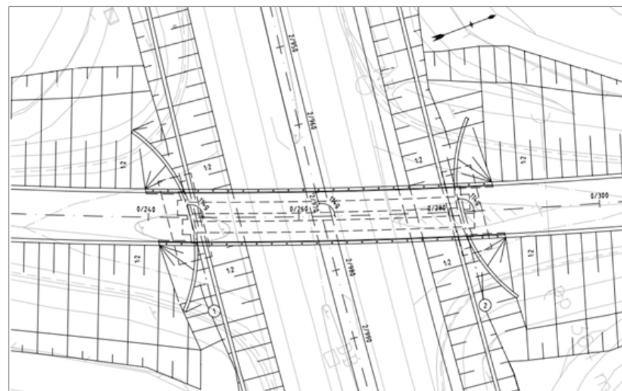
Figur 23. Plan alternativ 2 – Balkrambro med mjukt svängda vingmurar. Vingmurarna utformats med en genomgående konvex form i plan (radie 20 m). Lika som för trafikplats Vambåsa för att bidra till en sammanhållen gestaltning längs sträckan. PM byggnadsverk
