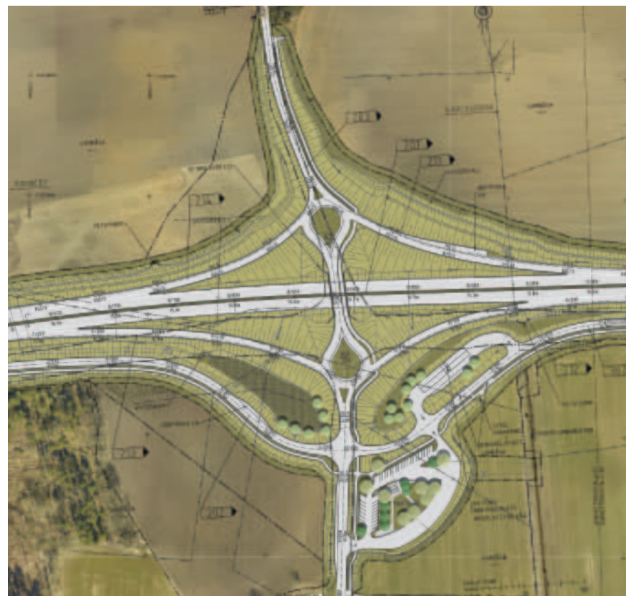
Figur 41. Illustration av Vambåsa trafikplats och rastplats: Nya träd har illustrerats vid dagvattenmagasin och trafikkontrollplats samt rastplats med pendelparkering.
