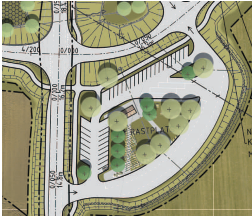
Figur 44. Illustration av rastplatsen med pendlarparkering: Rastplatsen ska likna en åkerholme med en upphöjd mitt. Stora träd omger en öppen glänta med plats för rörelse och lek. En tillgänglighetsanpassad servicebyggnad är placerad närmast pendlarparkeringen i norr. Gångvägar leder ut från servicebyggnaden. Sittbänkar har placerats nära gångarna. En pergola över den västra gången ger skugga till dess att träden växt sig stora. En stenmur avgränsar mot lastbilsparkeeringarna i söder och ramar in "åkerholmen".
