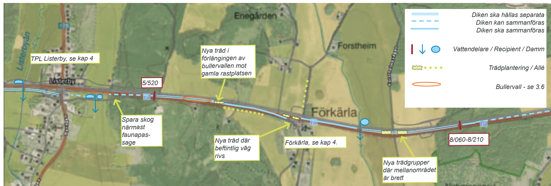
Översiktskarta 1b. Sidoområden, sträckan km 4/260 till km 8/560
