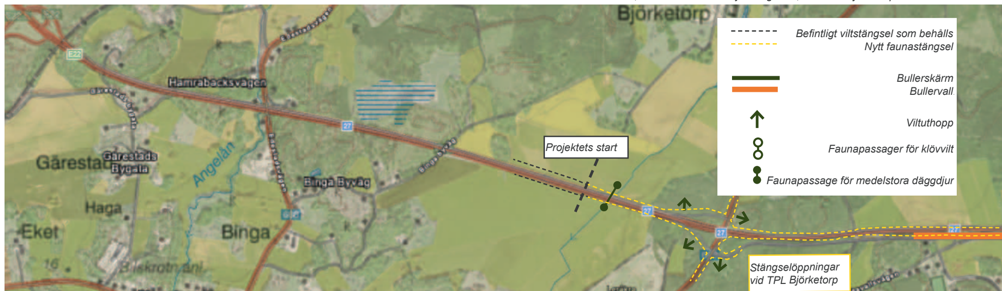
Översiktskarta 2a, Fauna- och bullerskyddsåtgärder, sträckan Björketorp till km 4/260
