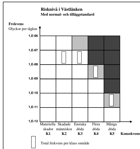
Figur 4 Riskmatris för Västlänkens tunnlar
