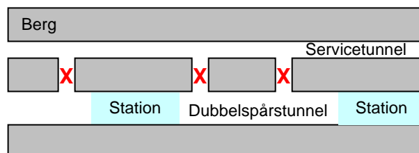
Figur 13 Brandsektionering mellan utrymmen
