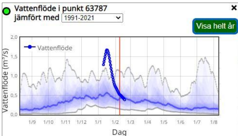
Figur 21 Vattenflödet i Knipån 1991-2021 (SMHI, Vattenweb)
