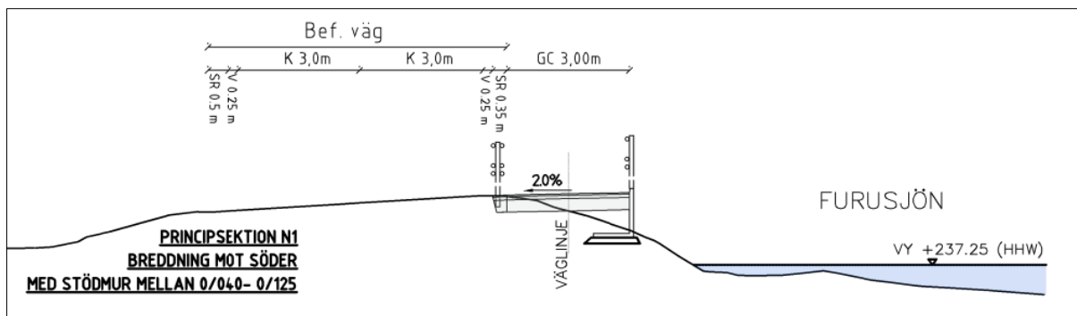
Figur 29 Sektion, cykelväg med stödmur mot Furusjön. Vattenyta vid högsta högvatten.
