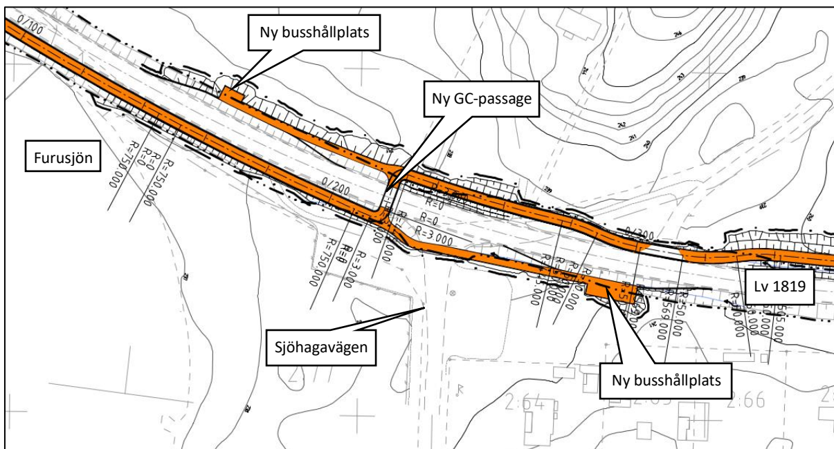
Figur 30 Föreslagen placering och utformning av gång- och cykelpassage vid Furusjö.
