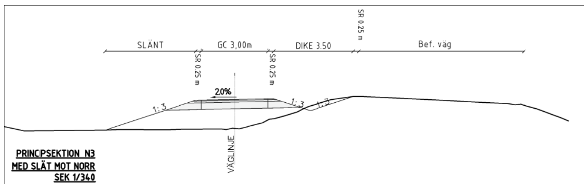
Figur 28 Sektion, exempel på sträcka där avvattning sker via gemensamt dike med länsväg 1819.
