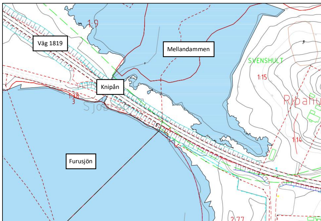
Figur 22 Vattenområde vid högsta högvatten (+237,25) i Furusjön, Mellandammen och Knipån i anslutning till länsväg 1819.
