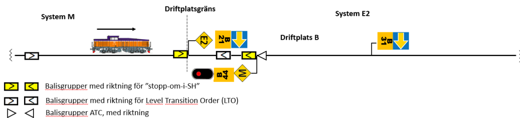
Bild 17. Färd från linjen i system M till driftplats i system E2 (exempel).
