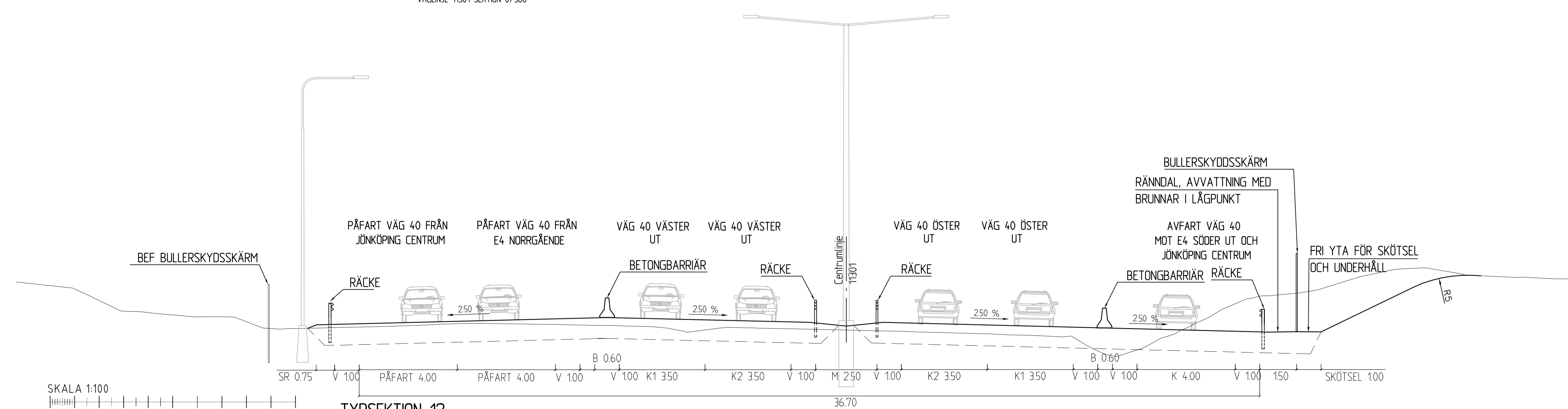
TYPSEKTION 12 VÄG 40 (BREDASTE SEKTIONEN VÄG 40 NÄRMOST VÄSTER OM TRAFIKPLATS LJUNGARUM) VÄGLINJE 11301 SEKTION 0/440
