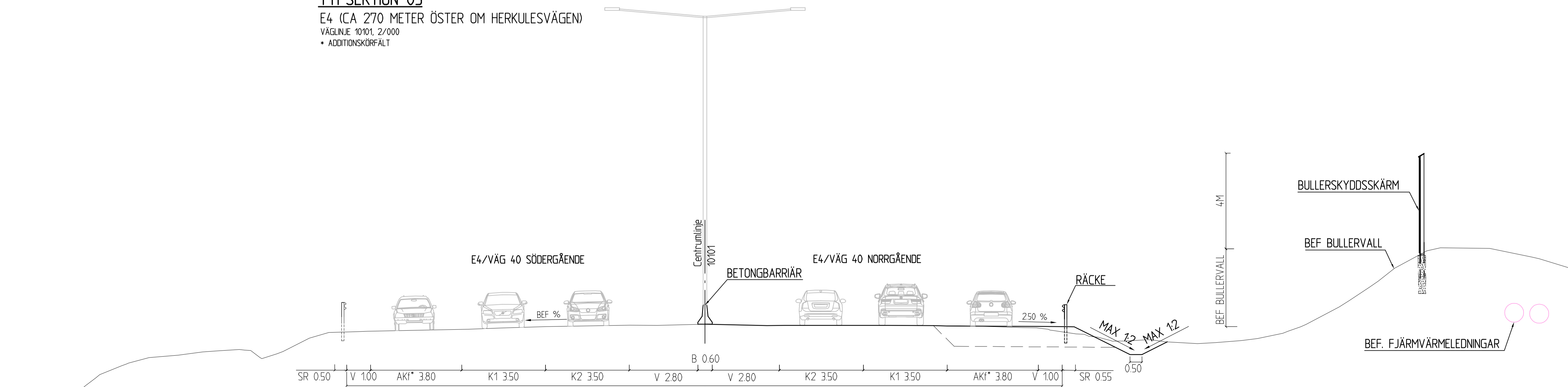
TYPSEKTION 06 E4 (CA 30 METER ÖSTER OM PORT MELLAN YTTRE LJUNGARUMSVÄGEN OCH SOLÅSEN) VÄGLINJE 10101, 2/430 • ADDITIONSKÖRFÄLT
