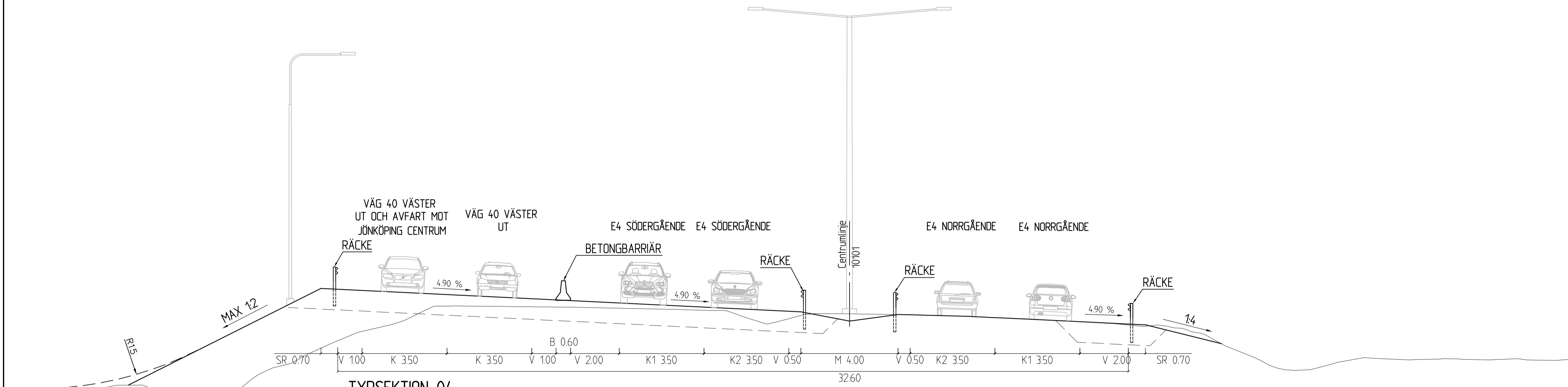
TYPSEKTION 04 E4 (CA 50 METER ÖSTER OM INDUSTRIGATAN) VÄGLINJE 10101, 1/400
