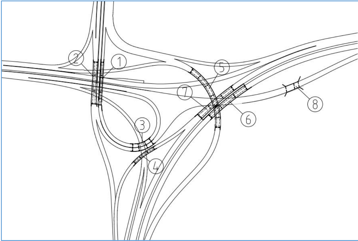
Figur 32. Översiktsplan över nya broar ingående i trafikplats Ljungarum.
