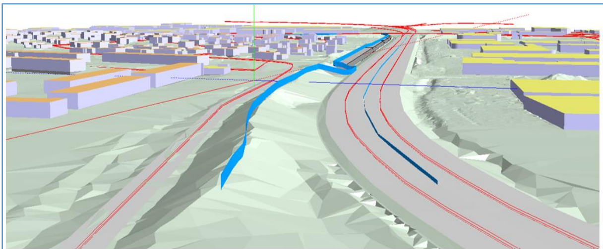
Figur 47. Föreslagna bullerskyddsåtgärder för delen efter Backen/Ljungarum fram till korsningen med Strömsbergsbäcken.
