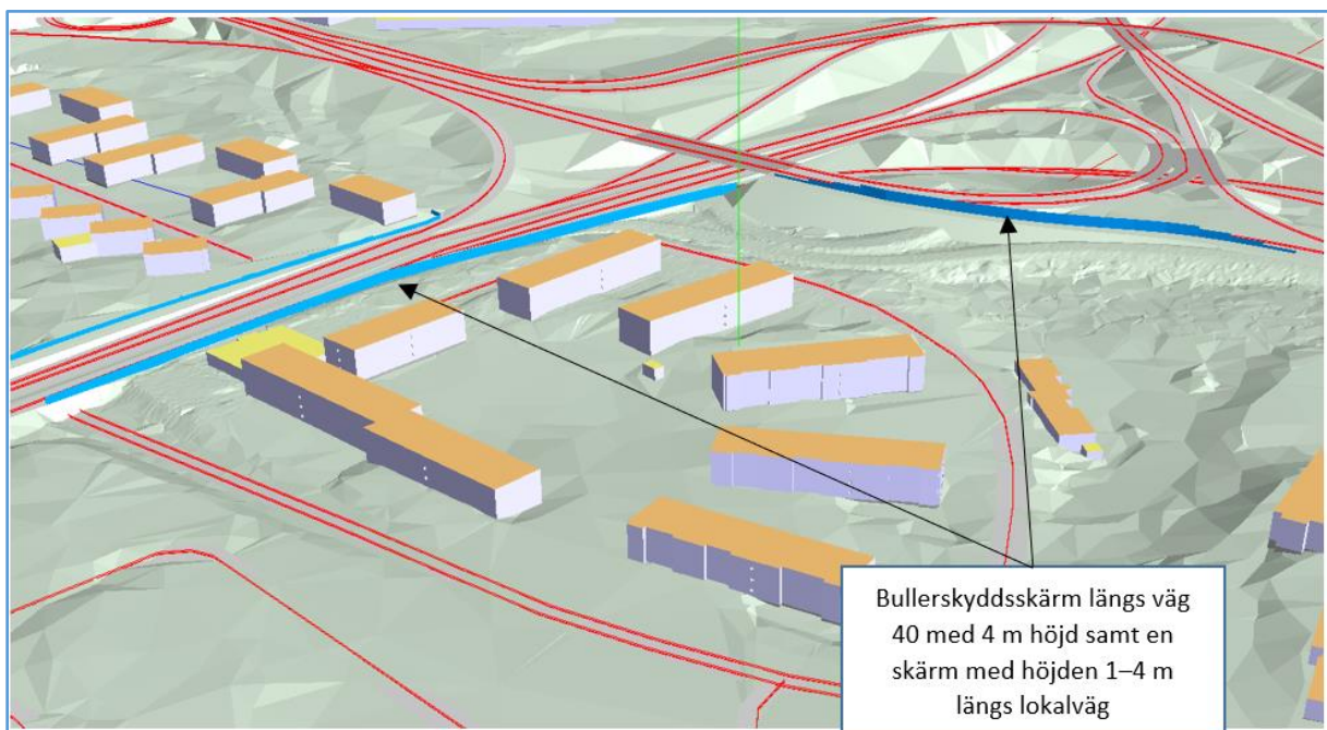
Figur 45. Föreslagna bullerskyddsåtgärder i anslutning till väg 40 och parallellkörbanan från Jönköpings centrum mot Råslätt.
