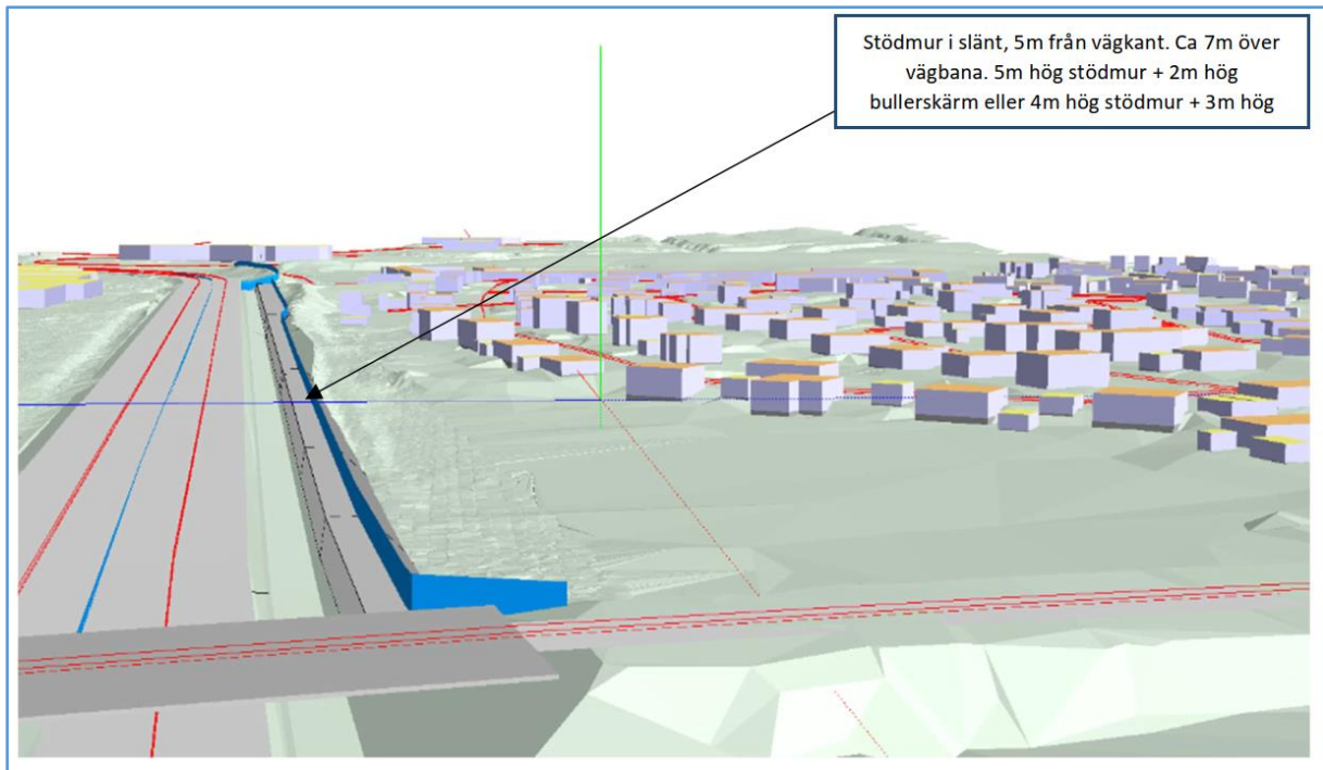
Figur 46. Föreslagna bullerskyddsåtgärder i anslutning till delen förbi Backen/Ljungarum.
