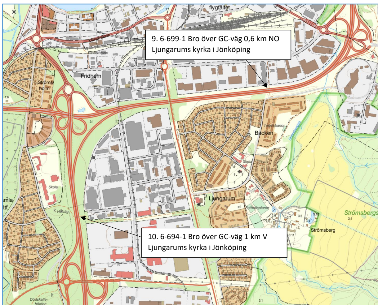
Figur 33. Befintliga GC-portar som kommer att breddas.
