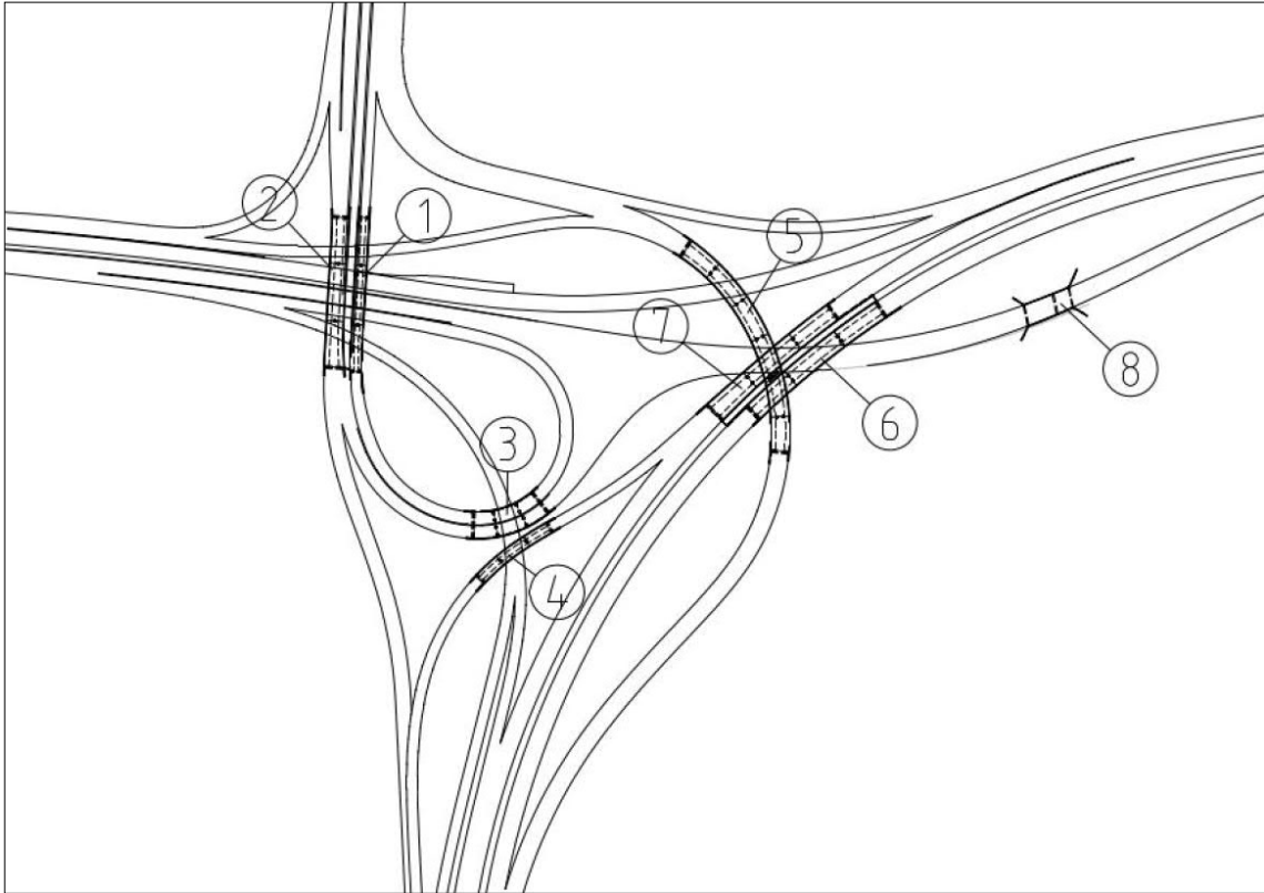
Figur 24. Mellanstöd för norra sidan av väg 40 för bro nummer 6 och 7 kommer att förläggas lägst inom trafikplatsen.
