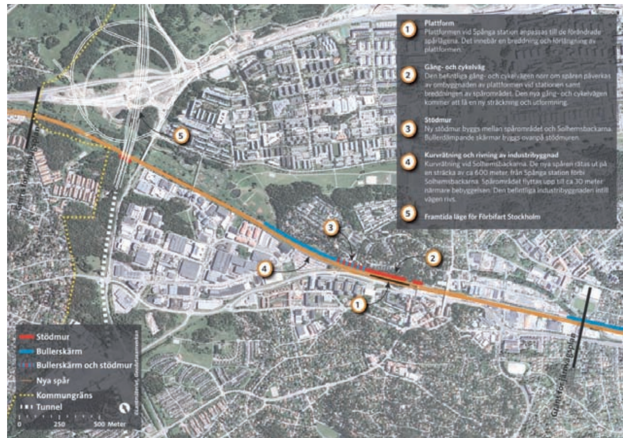
Figur 5. Översiktlig bild som visar spårutbyggnaden mellan Spånga och Barkarby. Obs: Bullerskärmarna på bilden kommer att tas bort för att stämma överens med MKBn.
