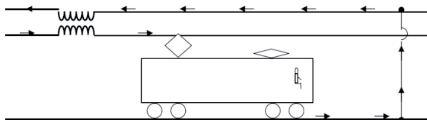
Figur 10. Strömmen matas via kontaktledning (1) till tågets strömavtagare (2). Strömmen går genom tågets motorer och leds tillbaka via hjulen till den ena av rälsens två rälsar, S-rälen (3). Ungefär var femte kilometer finns en jordförbindelse (4) där strömmen sugas till en återledare (5). Det som ser till att strömmen sugas upp från S-rälen är sugtransformatorn (6) som sitter inkopplad på kontaktledningen och återledaren.
