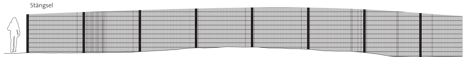
Figur 30. Princip för stängsel. Enligt AKJ är kravet minst 1,8 meter högt Skala 1:100
