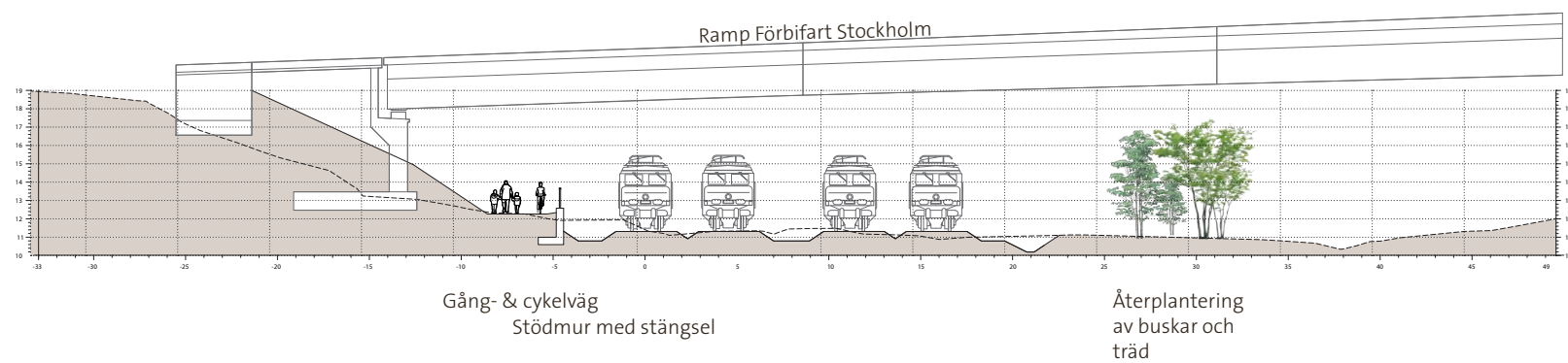
Figur 29. Sektion J-J, Km 13+260 Skala 1:400
