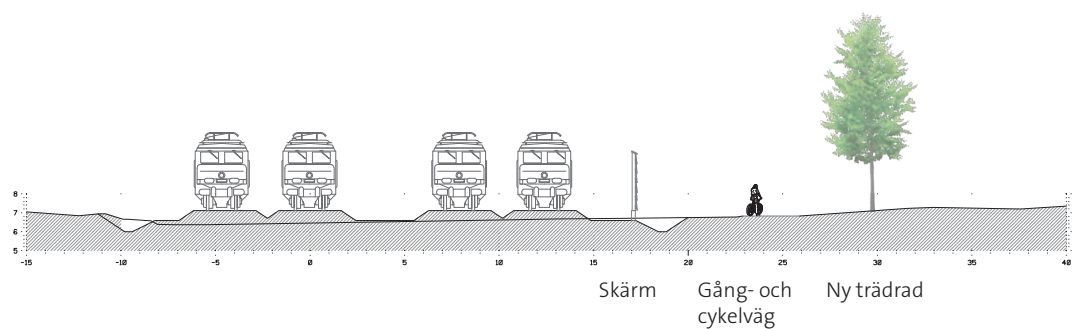
Figur 18. Sektion H-H, Km 11+930 Skala 1:400
