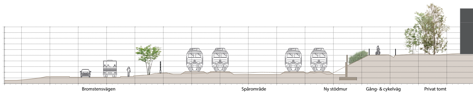
Figur 16. Sektion F-F, Km 11+650 Skala 1:400
