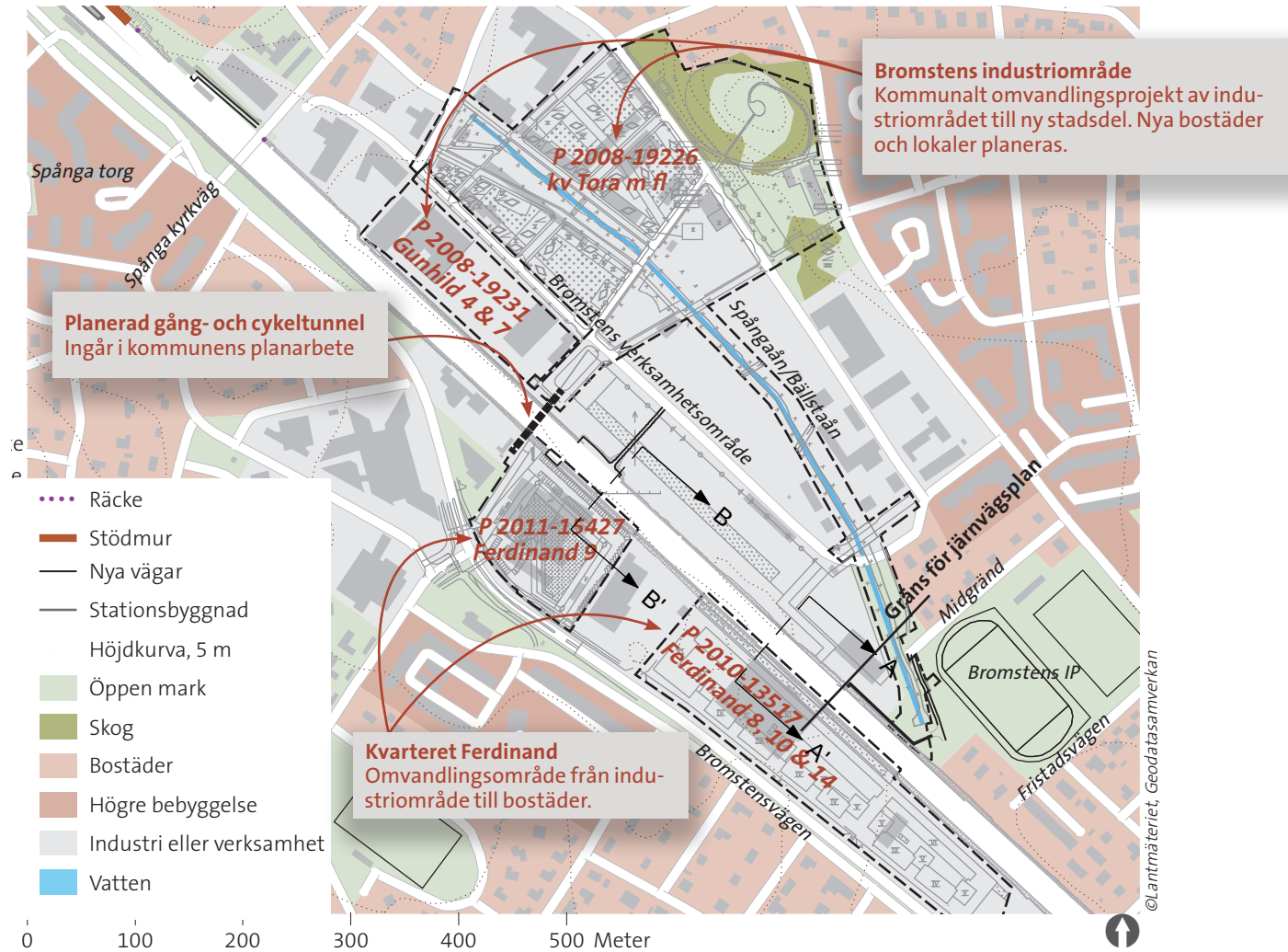
Figur 7. Övergripande plan för delsträckan Bromstens industriområde/kvarteret Ferdinand
