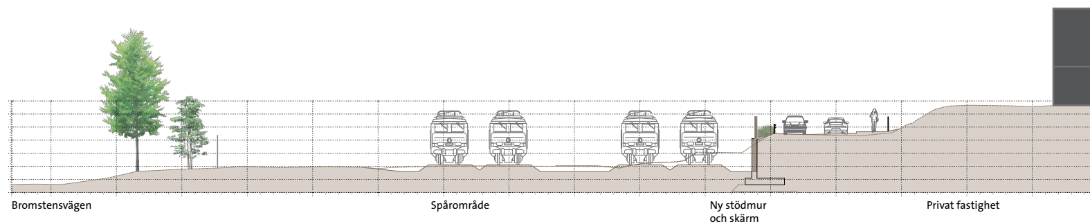
Figur 17. Sektion G-G, Km 11+740 Skala 1:400
