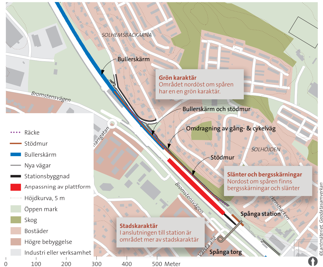
Figur 10. Övergripande plan för Spånga station/Solhöjden/Solhemsbackarna
