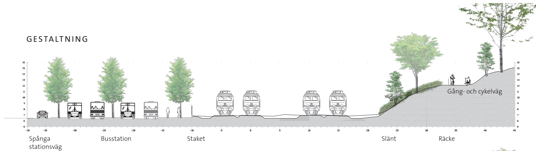
Figur 13. Sektion C-C, Km 11+200 Skala 1:400
