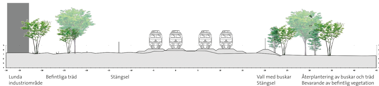
Figur 27. Sektion I-I, Km 12+675 Skala 1:400
