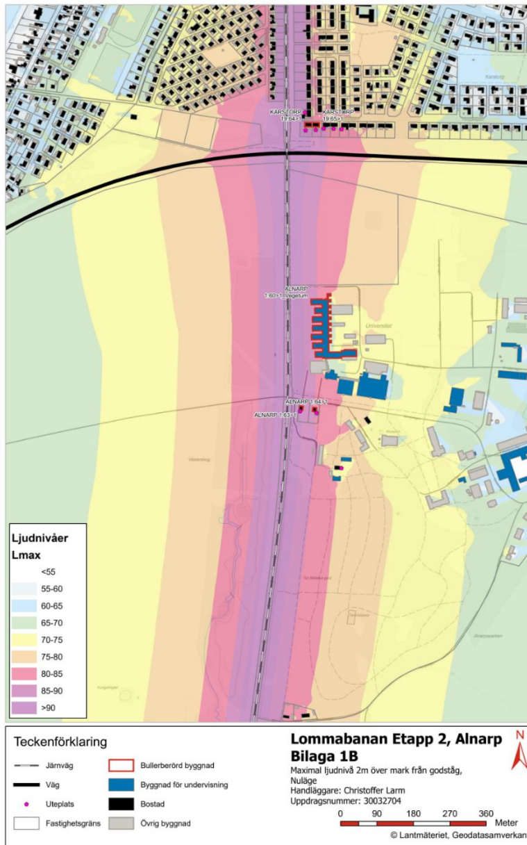
Figur 11. Bullerspridningskarta i nuläget för maximala ljudnivåer.
