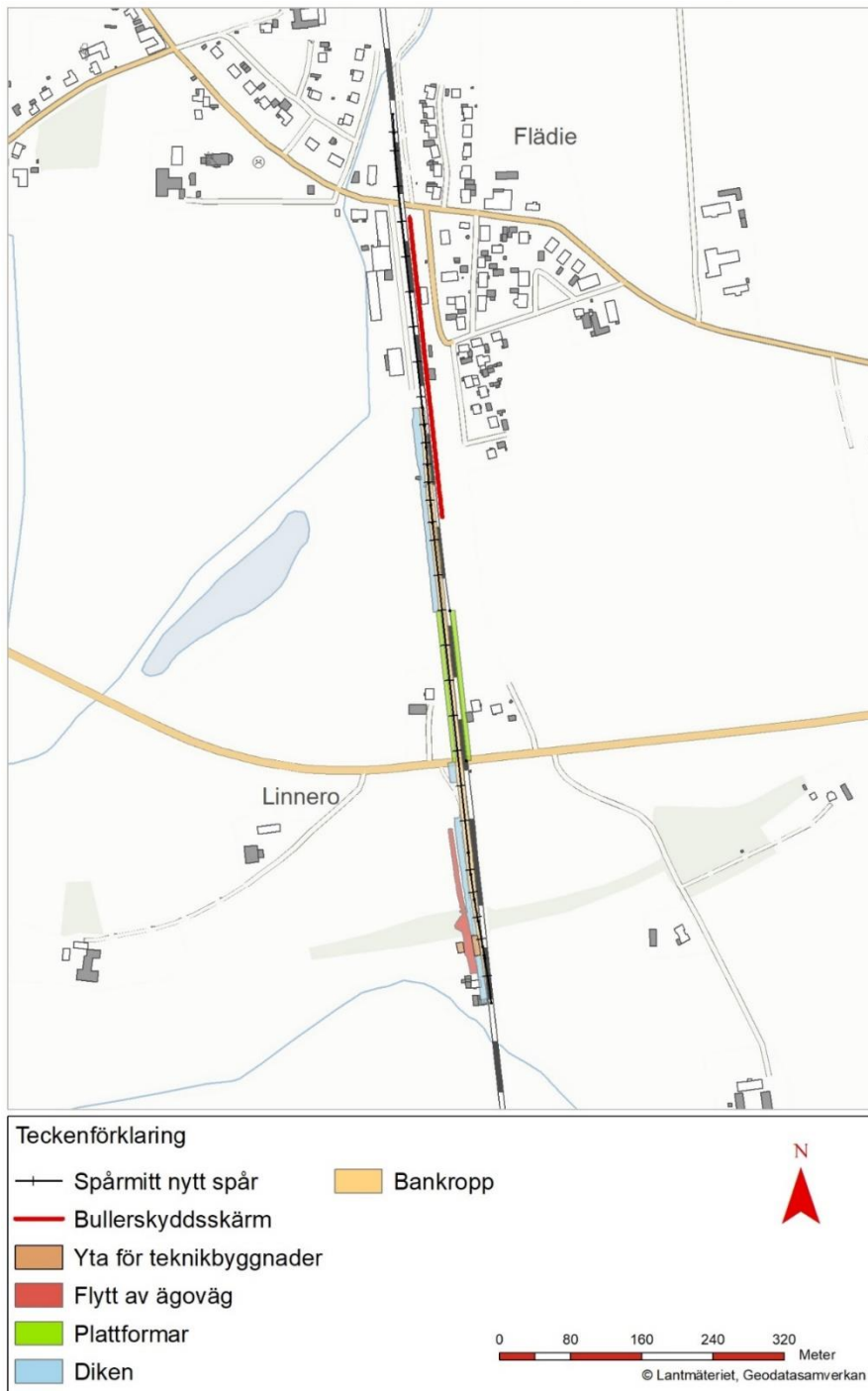
Figur 12. Placering av plattformar, teknikbyggnader och mötesspår (Sweco).
