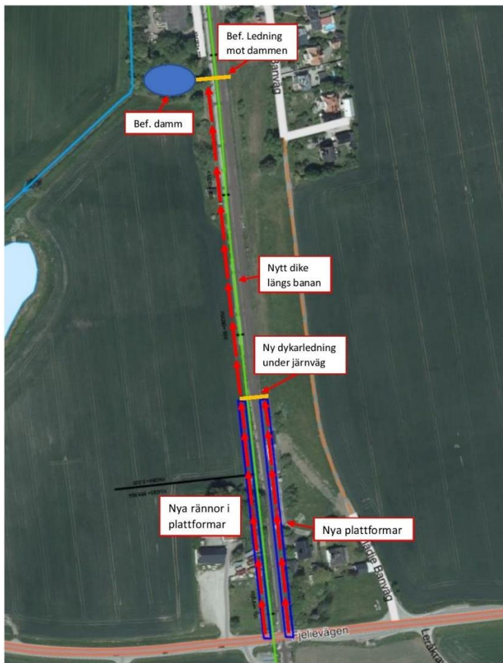
Figur 13. Befintliga dräneringssystem och principiella lösningar för dagvattenhanteringen i Flädie (norr om Fjellevägen) (Sweco).
