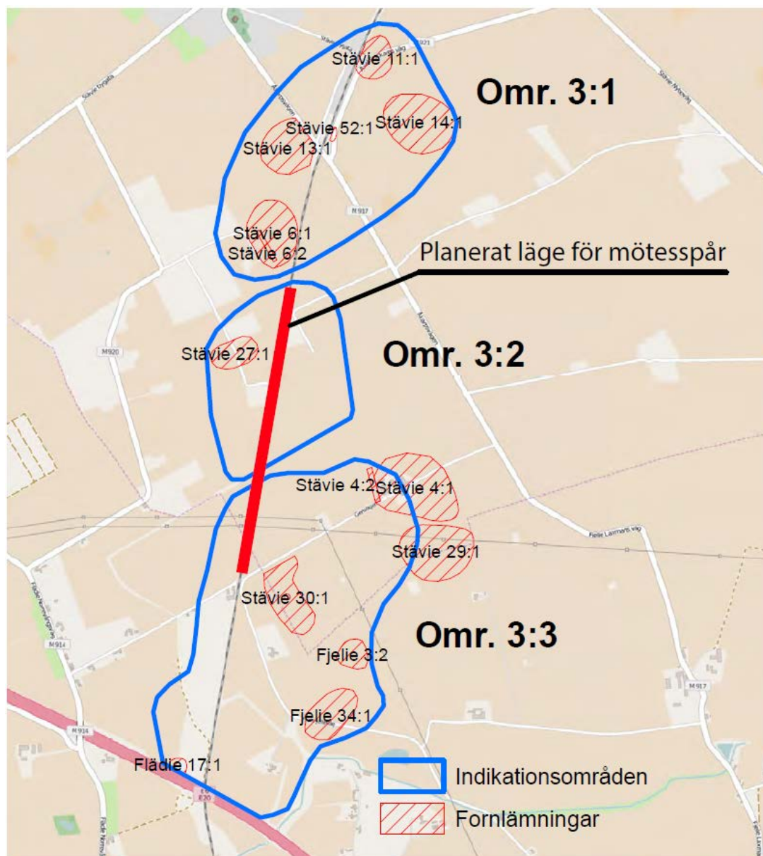
Figur 5.2:1 Karta över registrerade fornlämningar samt indikationsområden
