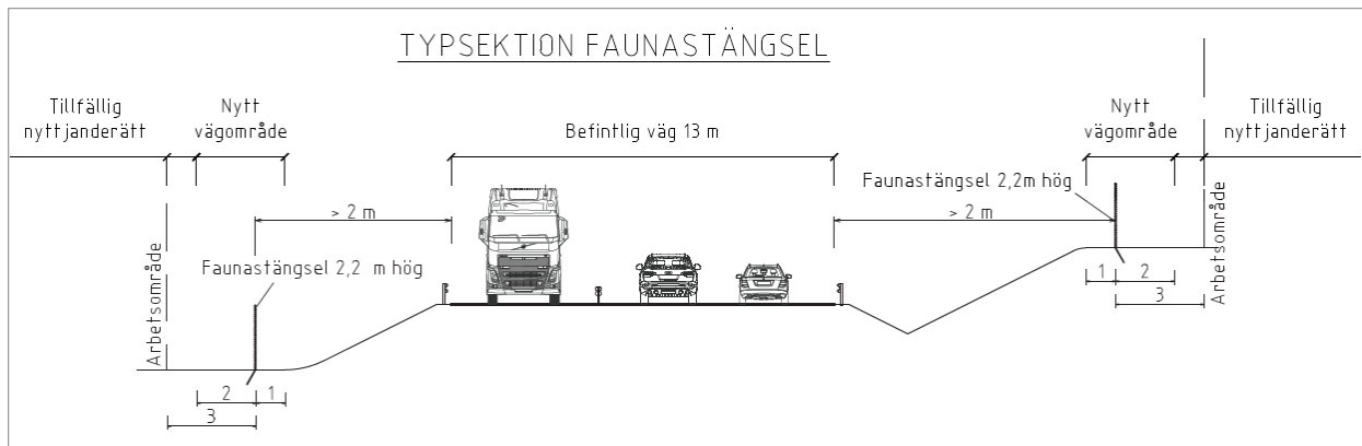
Figur 21. Principutförning för faunastängsel utmed väg 19 och 23.
