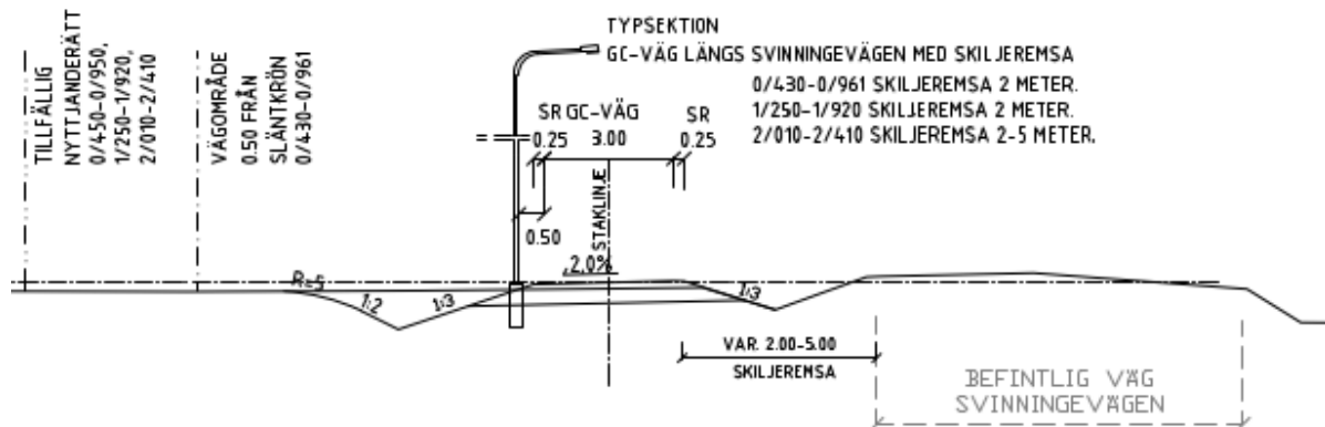
Figur 6. Sektion för gång- och cykelväg med skiljeremsa, ritning 132T0401.
