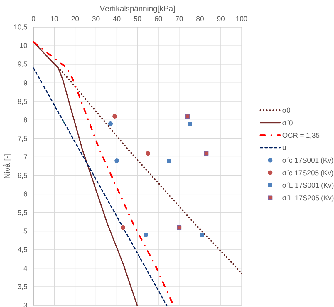
Figur 20. Spänningsdiagram Svinningevägen 0/840.
