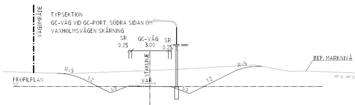
Figur 3. Sektion, gång- och cykelväg vid gång- och cykelport i skärning, ritning 131T0401.
