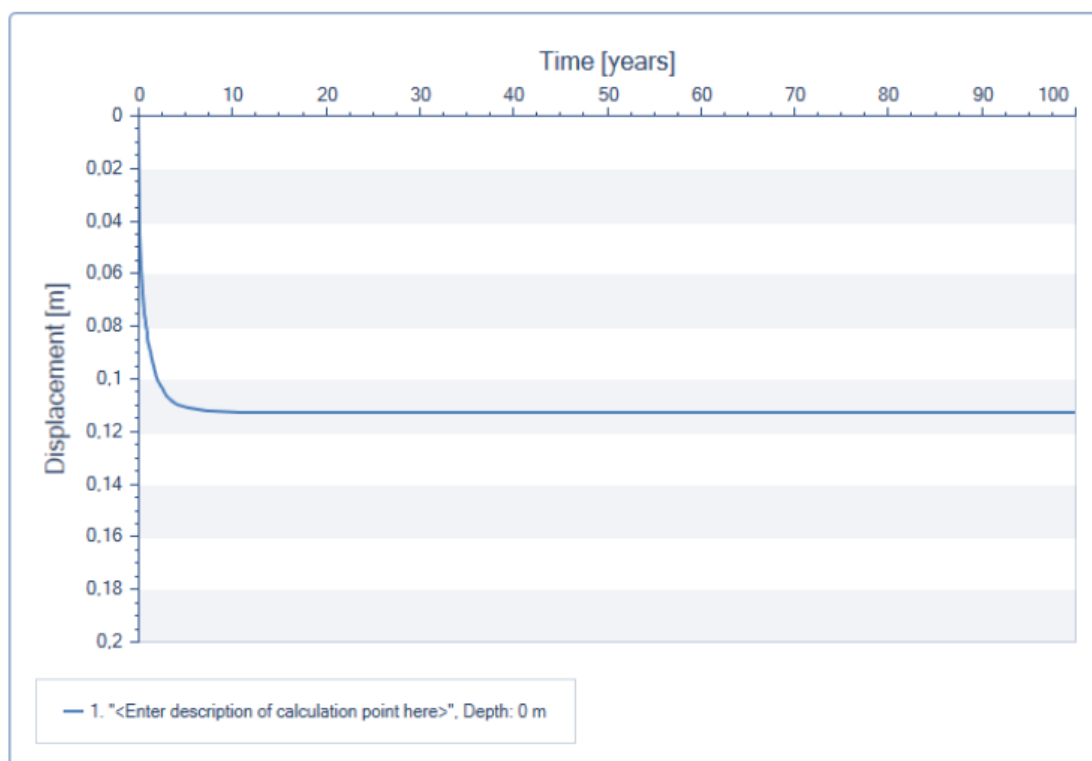
Figur 1 Sättningsberäkning för läge 1 med värden från 17S205/17S206B.
