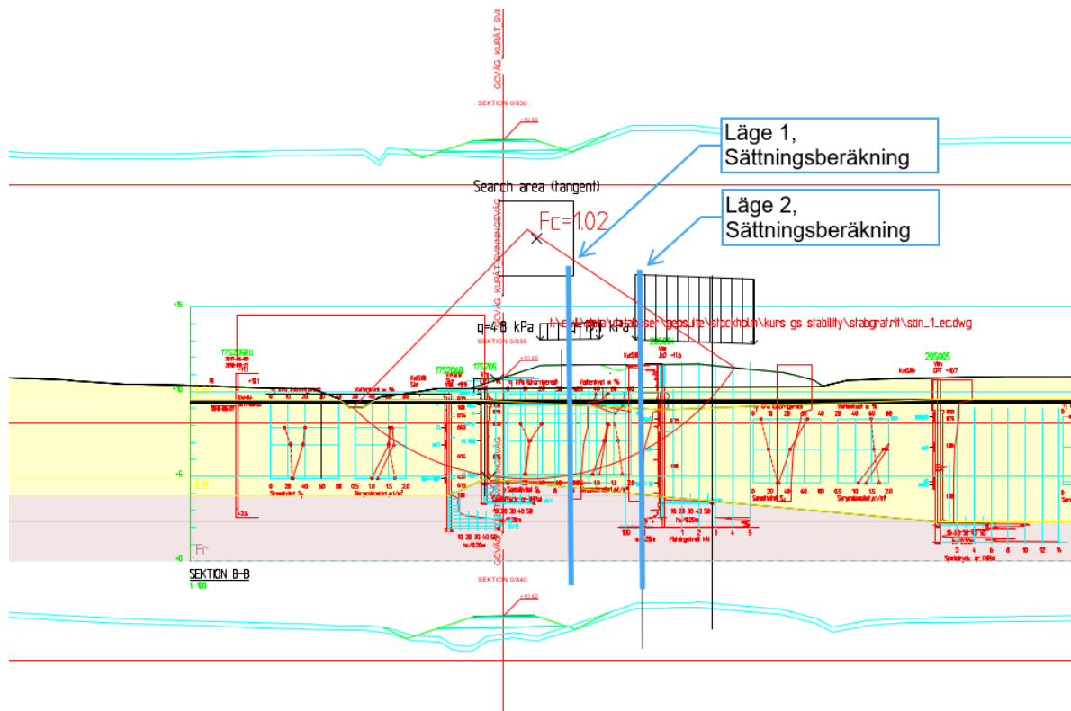
Sektion o/835 med planerad gång- cykelväg (partialkoefficientmetoden)
