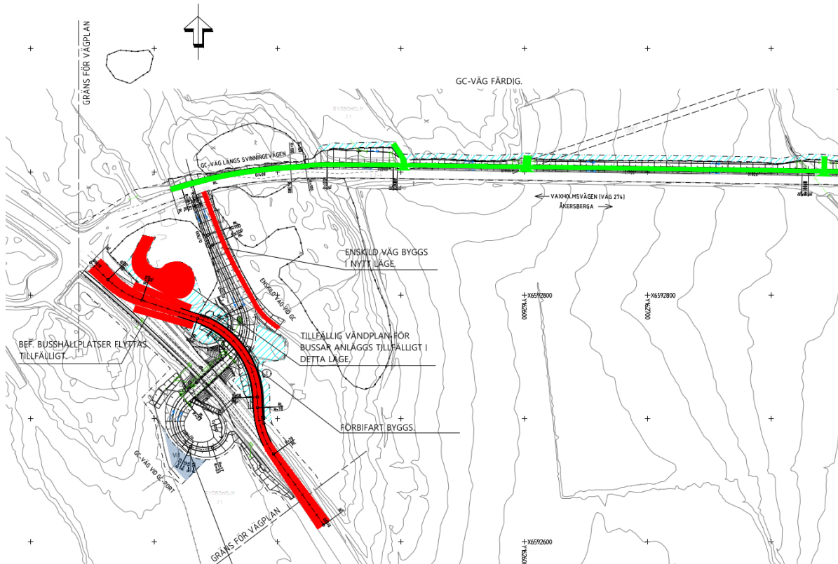
Figur 30. Skedesplan skede 3 TUB A, ritning 100T40A3.
