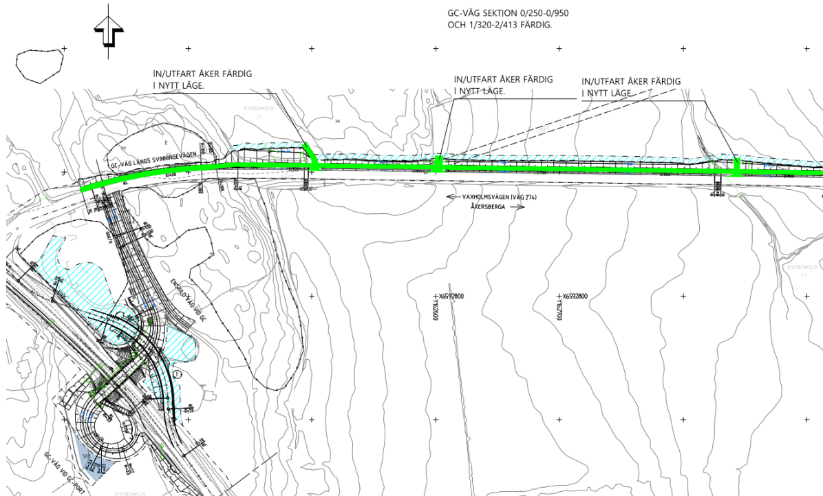
Figur 29. Skedesplan skede 2 TUB A, ritning 100T40A2.
