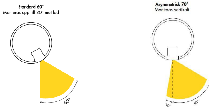
Figur 19 och 20. Illustration spridningsvinklar armatur HLS. Källa: Foxdesign.se
